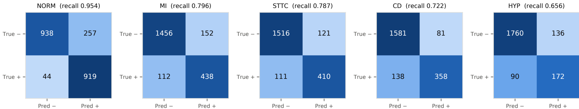
VOLT-KD (ours)
