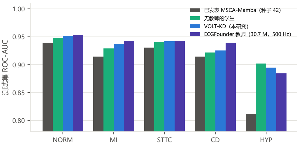
(a) 各类别区分能力
