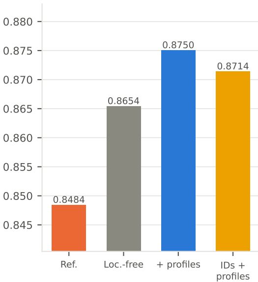
AUROC ↑
