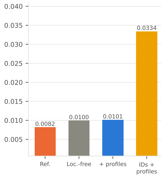
ICI ↓
