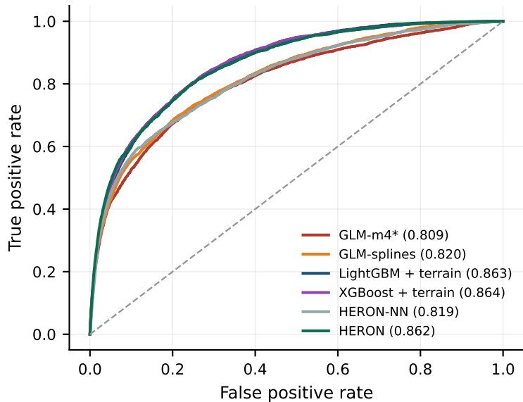
(a) ROC (AUC)
