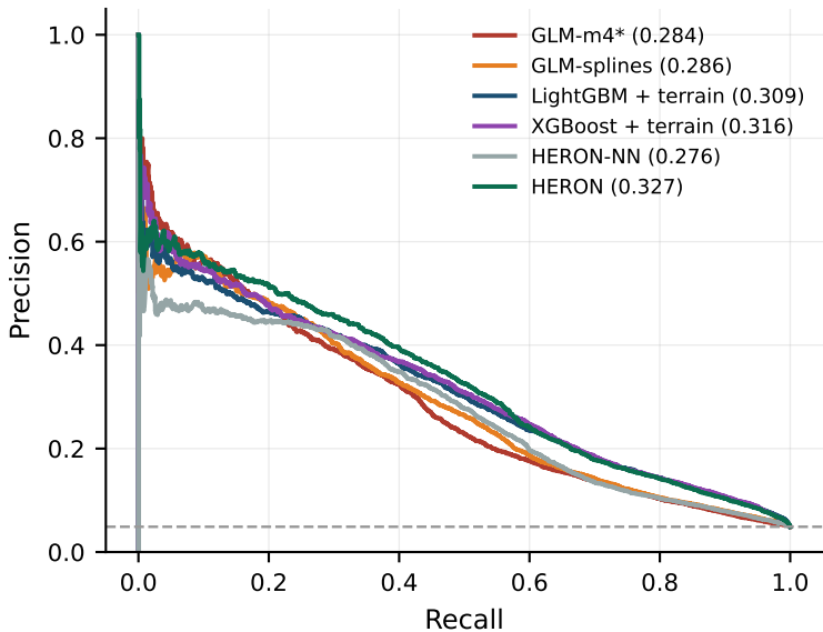
(b) Precision-recall (average precision)
