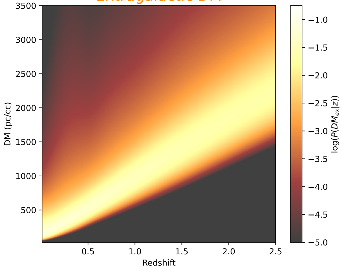
Extragalactic DM
