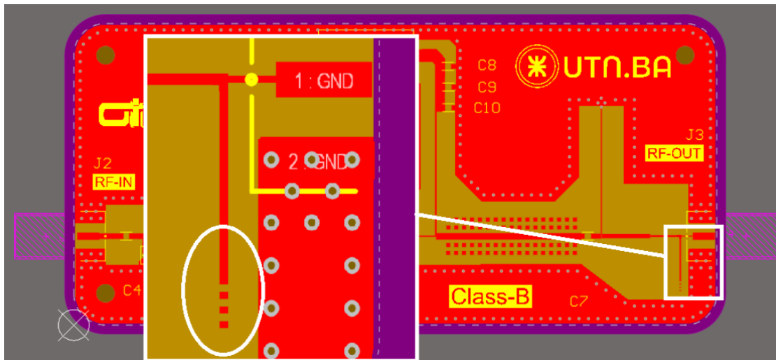
Figura 7.3: Pads adicionales incorporados para permitir la modificación del ancho de las líneas de transmisión, en caso de requerirse ajuste experimental.
