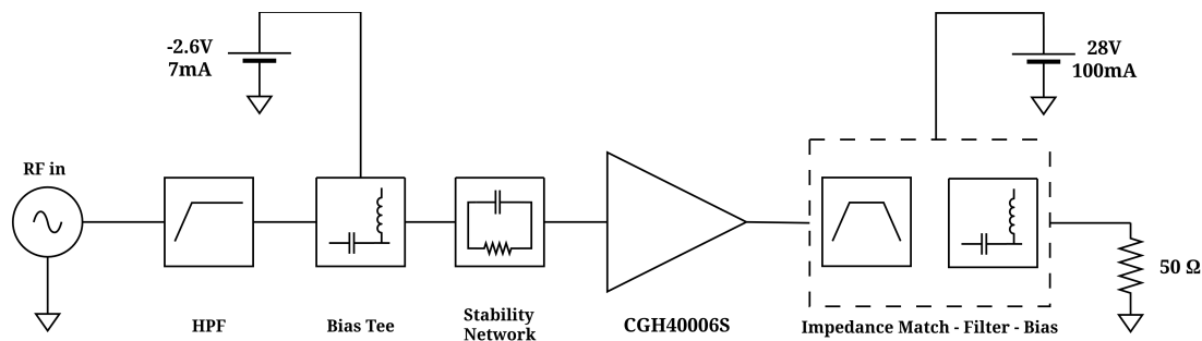
Figura 7.1: Diagrama en bloques de la topología propuesta para el amplificador de potencia.
