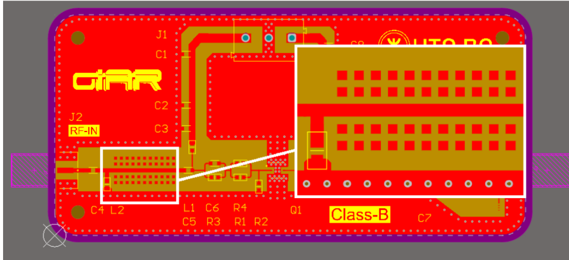
Figura 7.2: Pads adicionales incorporados para permitir la extensión de la longitud de los stubs de adaptación, en caso de requerirse ajuste experimental.
