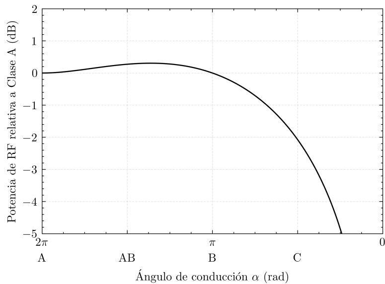
Figura 3.5: Potencia de RF entregada a la carga, relativa a Clase A, en función del ángulo de conducción, asumiendo carga óptima y cortocircuito en las frecuencias armónicas.
