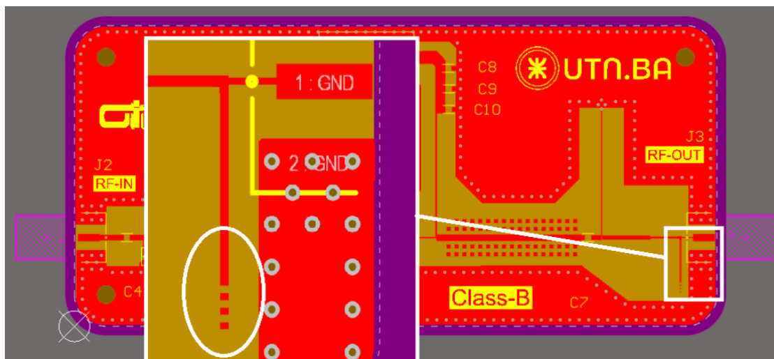
Figura 6.3: Pads adicionales incorporados para permitir la modificación del ancho de las líneas de transmisión, en caso de requerirse ajuste experimental.
