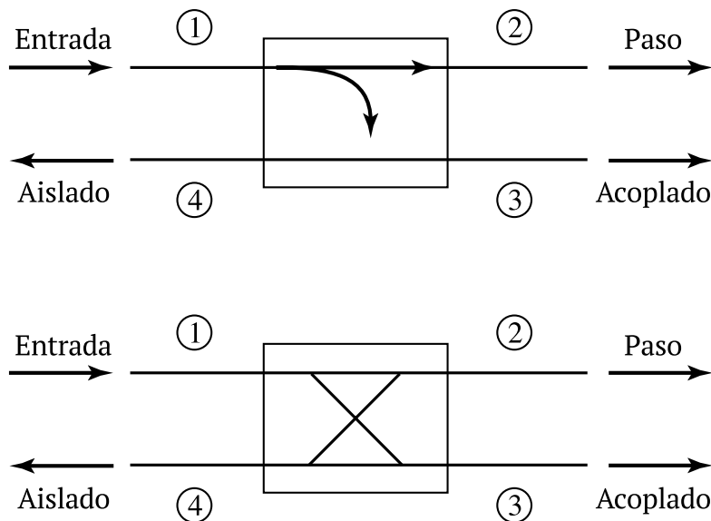
Figura 5.1: Dos símbolos comúnmente utilizados para acopladores direccionales.
