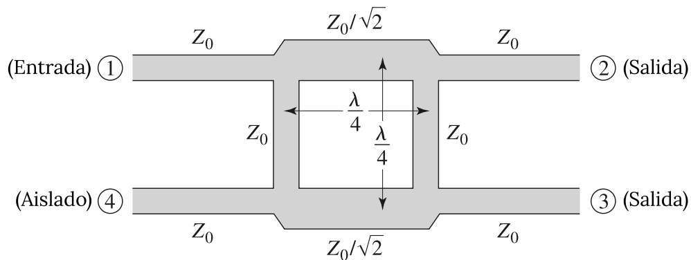
Figura 5.2: Geometría de un acoplador de línea ramificada.
