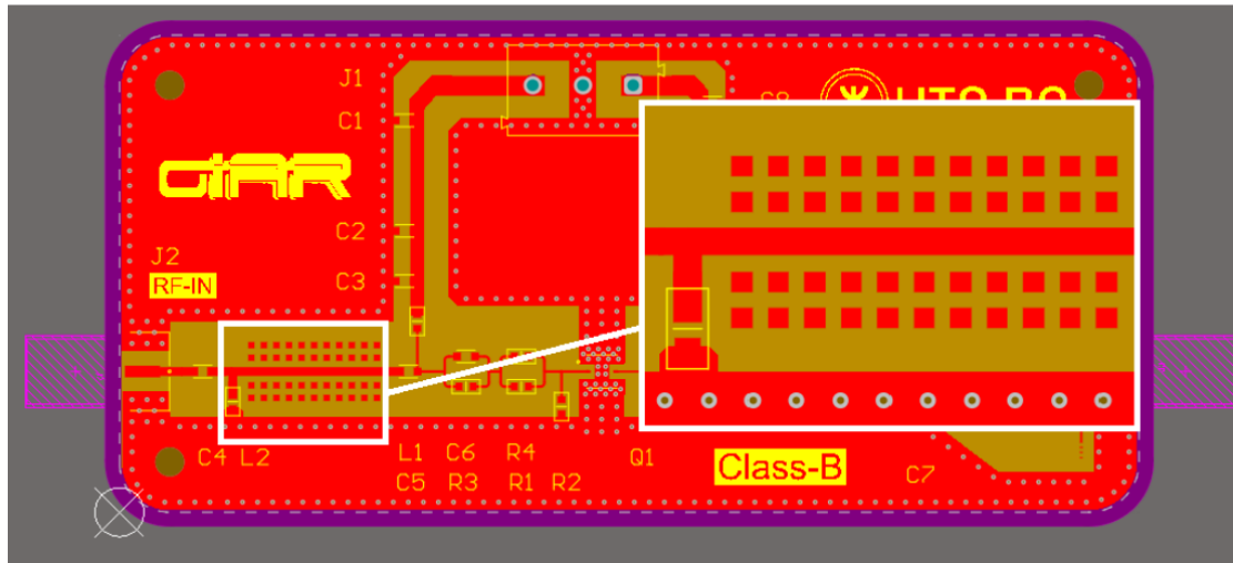
Figura 6.2: Pads adicionales incorporados para permitir la extensión de la longitud de los stubs de adaptación, en caso de requerirse ajuste experimental.
