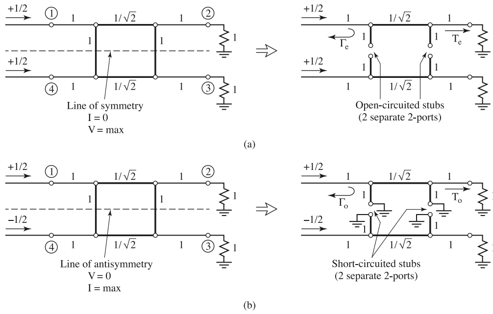
Figura 5.4: Descomposición del acoplador de línea ramificada en excitaciones de modo par e impar. (a) Modo par (e). (b) Modo impar (o).
