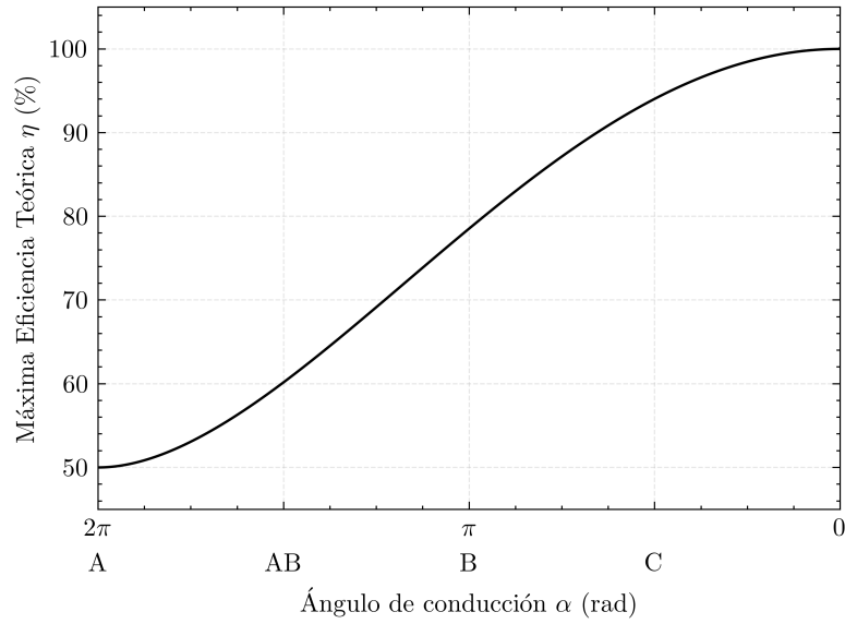
Figura 3.4: Eficiencia de drain teórica en función del ángulo de conducción, con las regiones correspondientes a las Clases A, AB, B y C señaladas.
