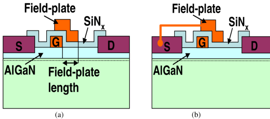
Figura 4.2: Sección transversal de las configuraciones de field plate conectado (a) al gate y (b) al source [33].
