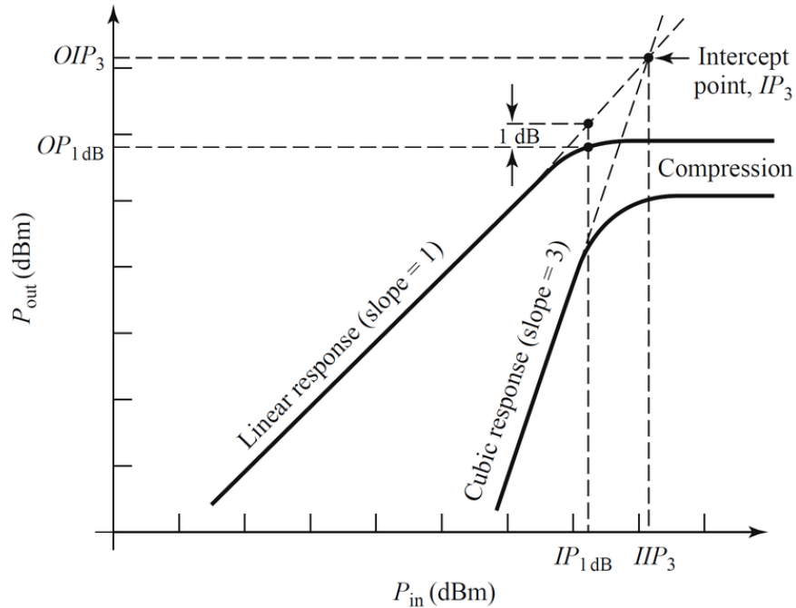
Figura 3.9: Curva teórica del punto de intercepción de tercer orden referido a la salida y del punto de compresión de 1 dB [30].
