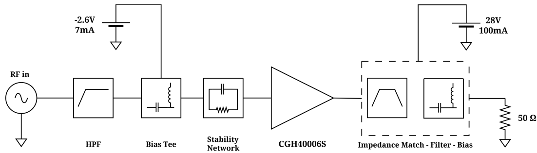
Figura 6.1: Diagrama en bloques de la topología propuesta para el amplificador de potencia.
