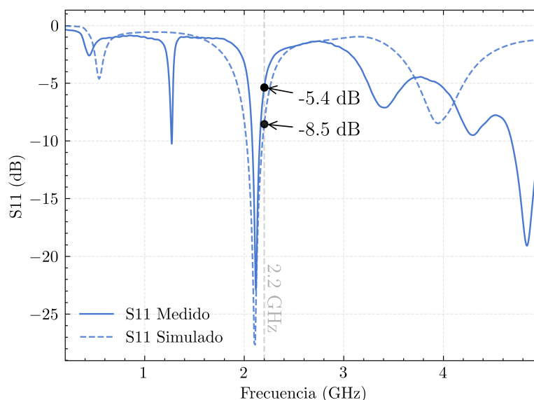
Figura 7.1: Comparación entre el S_{11} simulado (línea punteada) y medido (línea sólida) del amplificador de potencia fabricado.
