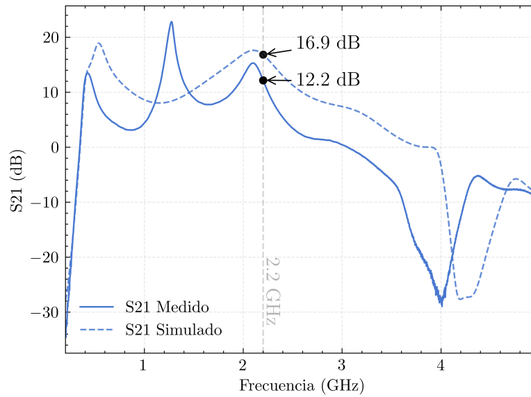
Figura 7.2: Comparación entre el S_{21} simulado (línea punteada) y medido (línea sólida) del amplificador de potencia fabricado.
