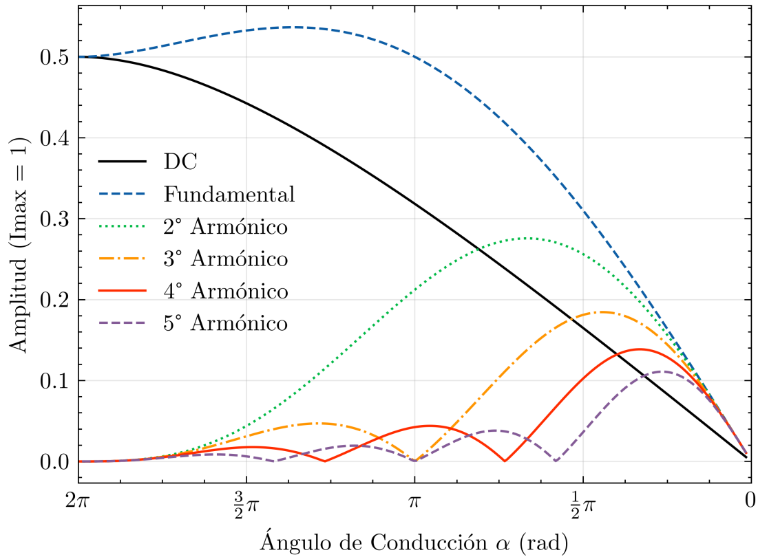
Figura 3.3: Amplitud normalizada de las componentes I_{DC} a I_5 de la corriente de drain en función del ángulo de conducción \alpha .
