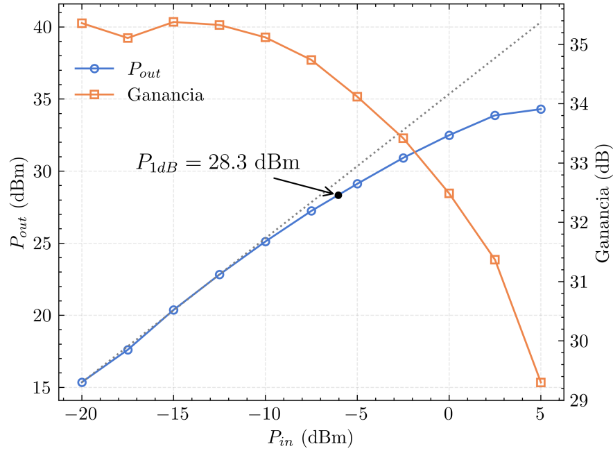
Figura 7.3: Potencia de salida medida (azul) y ganancia (naranja) en función de la potencia de entrada para la cadena driver-DUT. La línea punteada gris representa la característica de transferencia lineal ideal obtenida de la extrapolación de ganancia de pequeña señal.
