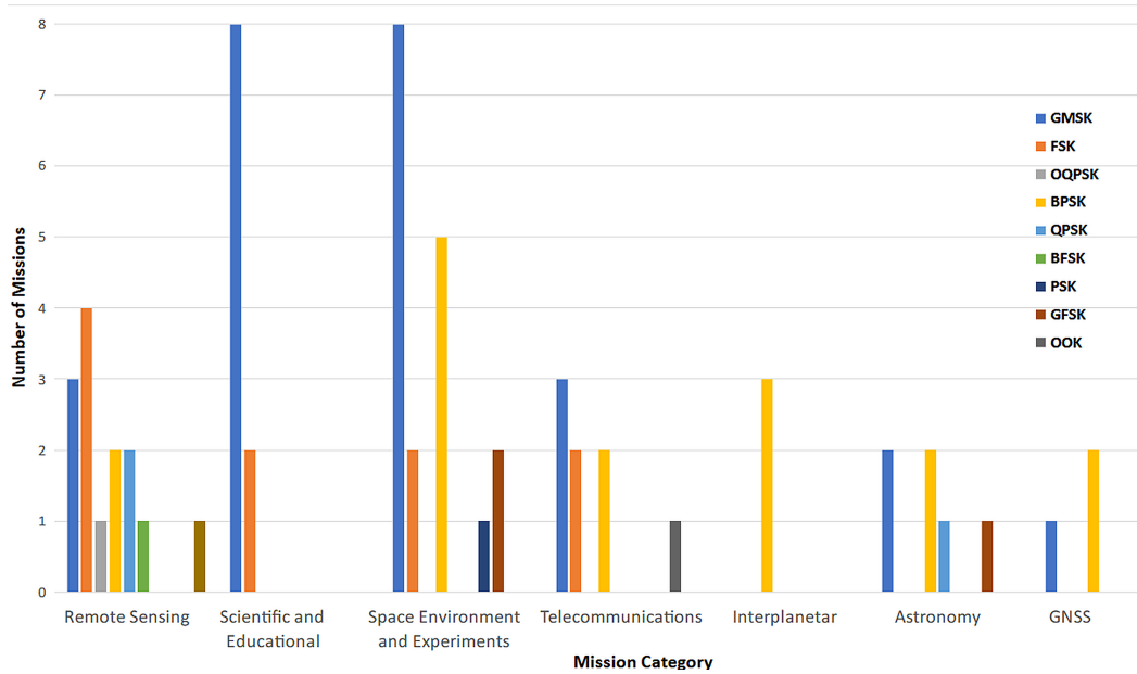
Figura 2.3: Distribución de esquemas de modulación empleados en misiones CubeSat, discriminada por categoría de misión. Adaptado de [4].
