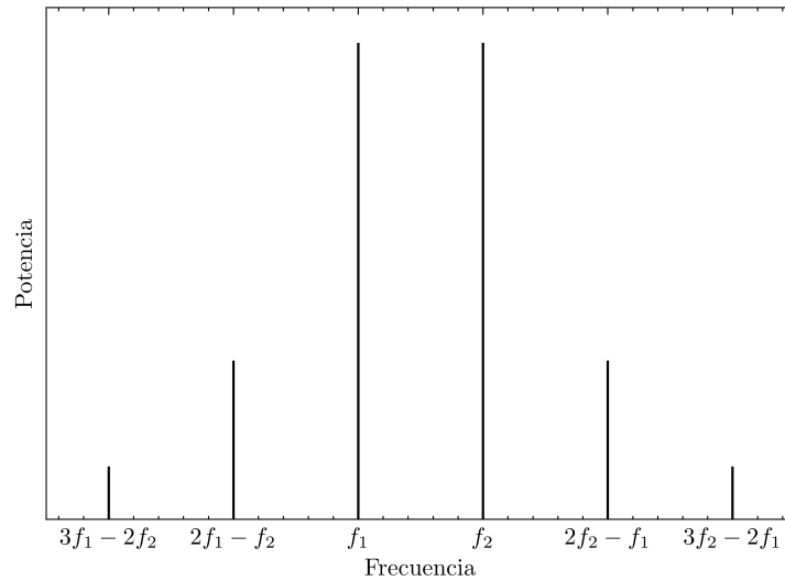
Figura 3.8: Productos de intermodulación cercanos a las frecuencias de los tonos de la señal de entrada.
