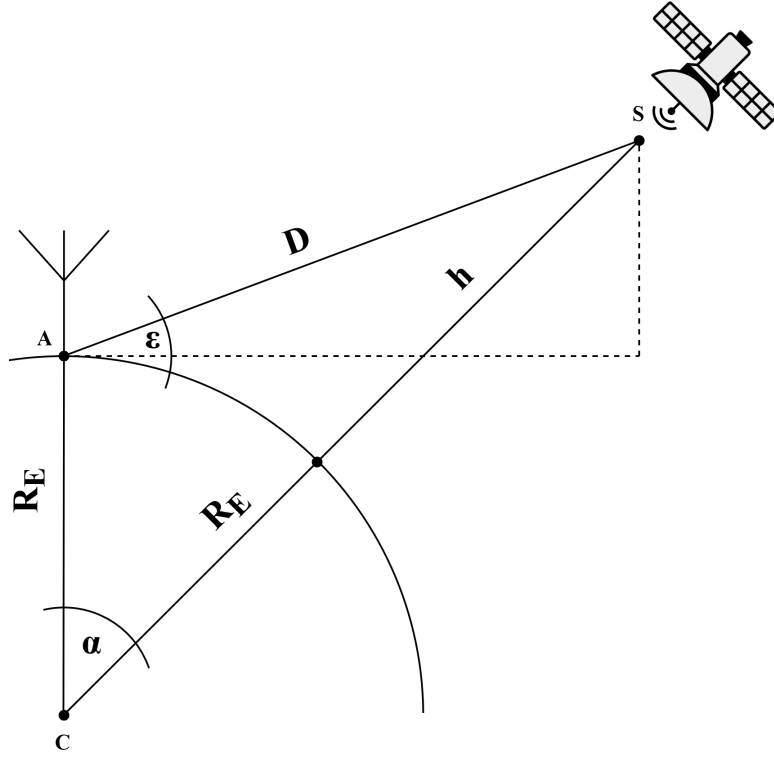
Figura 6.4: Modelo matemático para el cálculo de la distancia D en función del ángulo de elevación \epsilon .
