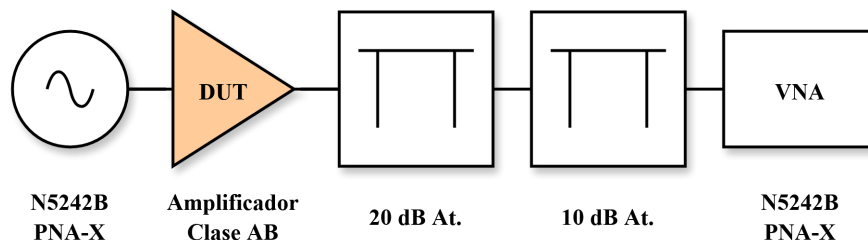
Figura 7.2: Diagrama en bloques del setup de medición de parámetros dispersión del amplificador.
