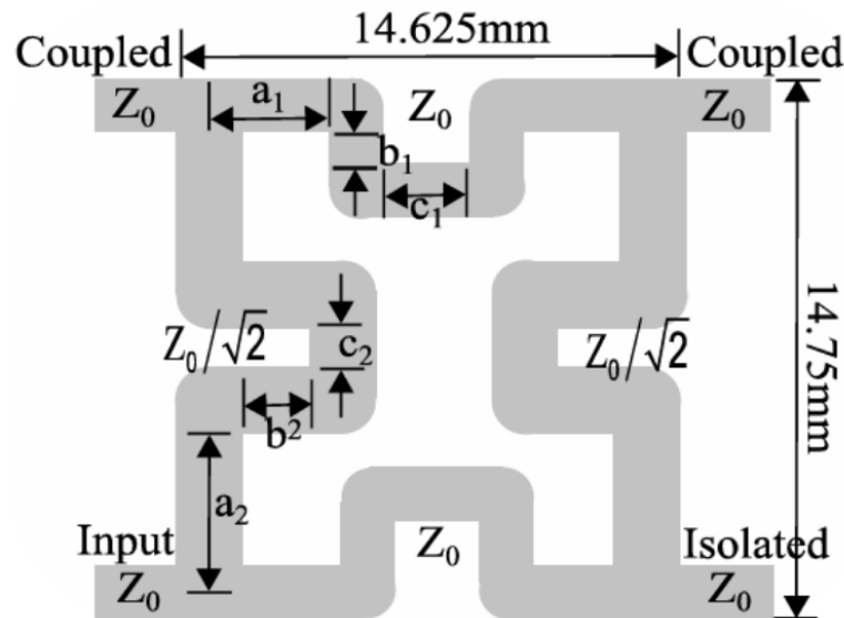
Figura 7.6: Parametrización de la topología plegada del acoplador mediante las variables geométricas a , b y c de cada tramo [47].
