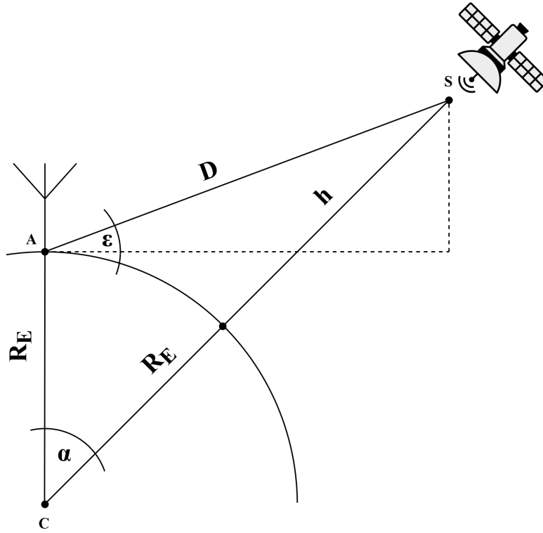
Figura 7.13: Modelo matemático para el cálculo de la distancia D en función del ángulo de elevación \epsilon ( \epsilon ).
