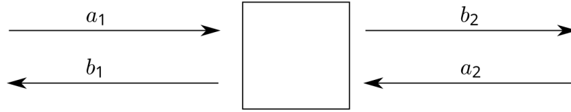
Figura 4.6: Cuadripolo genérico de dos puertos con sus ondas incidentes y reflejadas [26].
