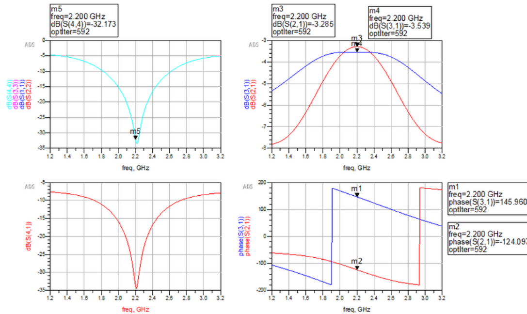
Figura 7.8: Parámetros de dispersión simulados del acoplador a nivel esquemático en ADS, luego de la optimización.
