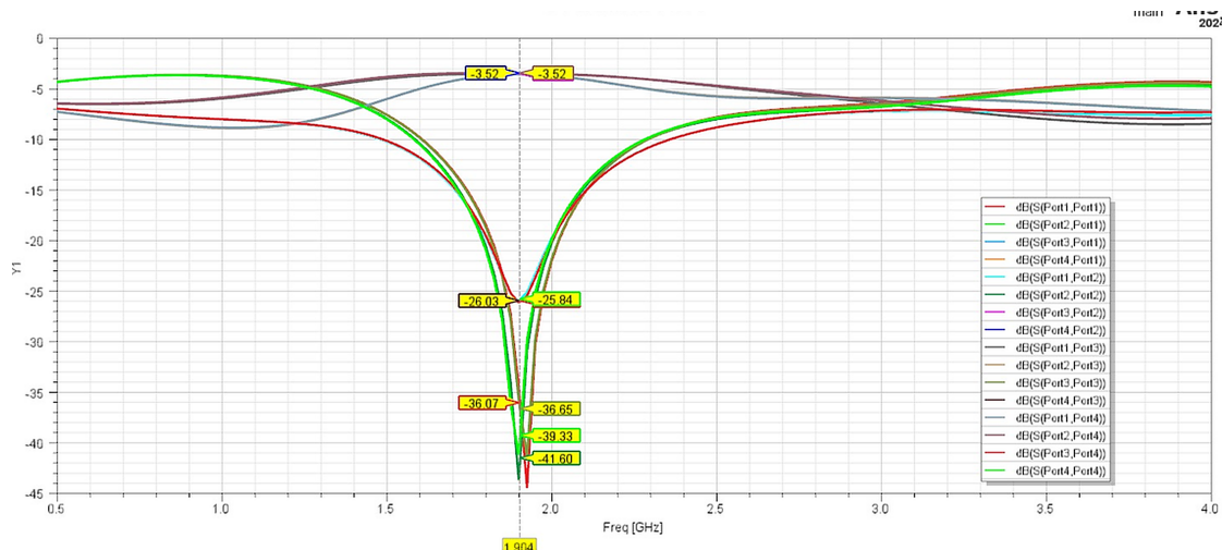
Figura 7.9: Parámetros de dispersión simulados en HFSS con el corrimiento de frecuencia observado.
