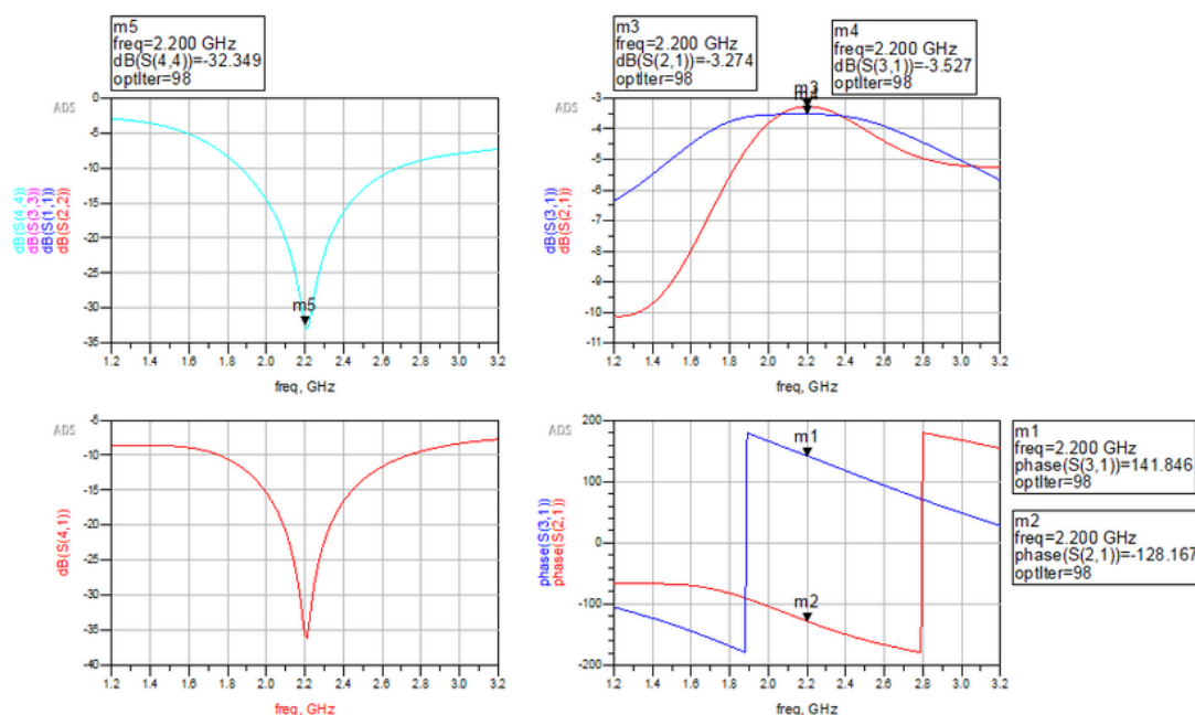
Figura 7.11: Parámetros de dispersión simulados del acoplador v2, incluyendo el modelado del pad de conexión SMA, luego de la reoptimización.
