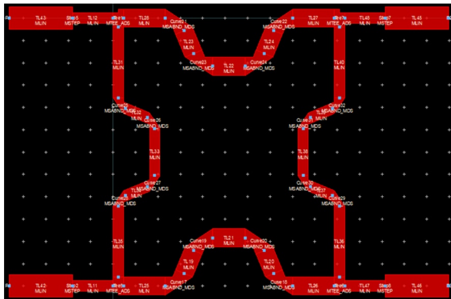
Figura 7.10: Layout del acoplador híbrido en ADS (acoplador v2).
