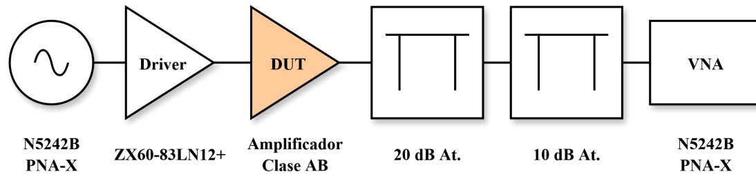
Figura 7.5: Diagrama en bloques del setup de medición de OIP3 del amplificador.
