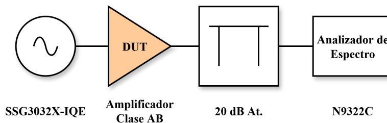
Figura 7.4: Diagrama en bloques del setup de medición de distorsión armónica del amplificador.
