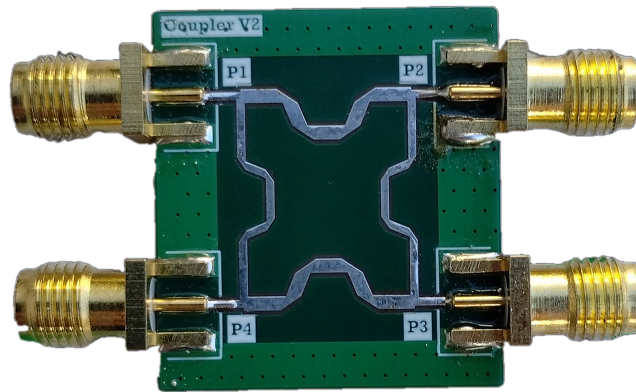
Figura 7.12: Placa de circuito impreso del acoplador v2.
