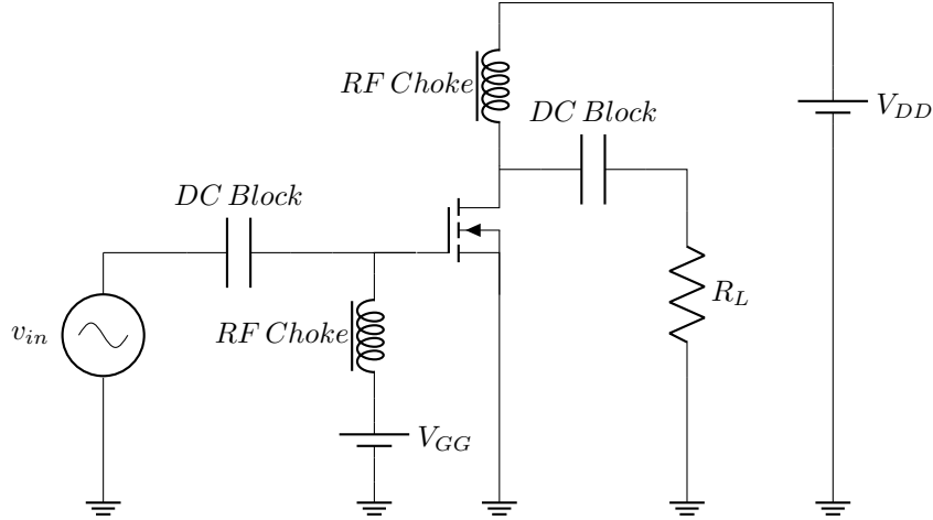
Figura 1: Esquema simplificado de una etapa de amplificación de radiofrecuencia con redes de polarización independientes de gate ( V_{GG} ) y drain ( V_{DD} ), utilizado como referencia para el análisis del ángulo de conducción.
