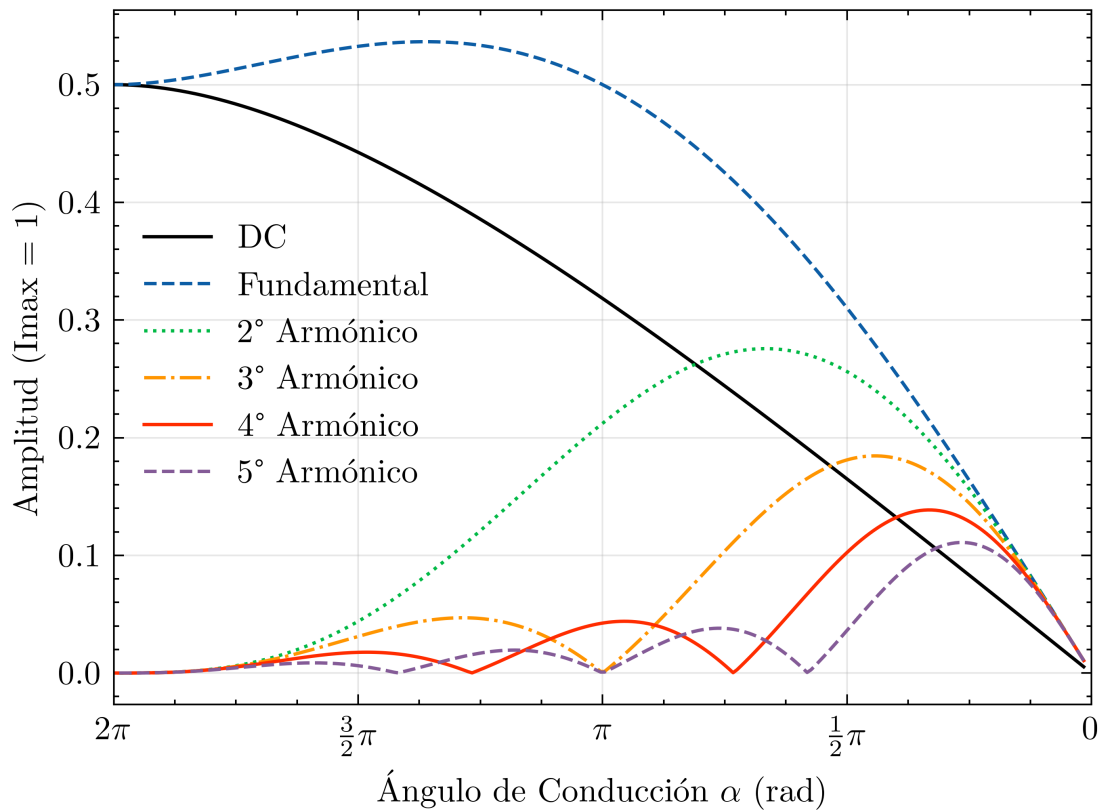
Figura 2.1: Amplitud normalizada de las componentes I_{dc} a I_5 de la corriente de drain en función del ángulo de conducción \alpha .
