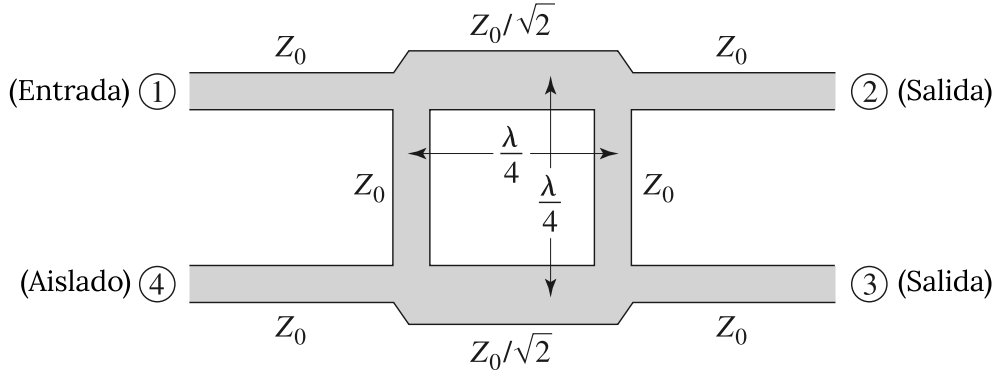
Figura 4.2: Geometría de un acoplador de línea ramificada.
