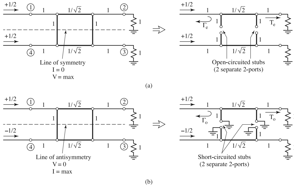
Figura 4.4: Descomposición del acoplador de línea ramificada en excitaciones de modo par e impar. (a) Modo par (e). (b) Modo impar (o).
