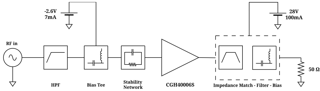
Figura 5.1: Diagrama en bloques de la topología propuesta para el amplificador de potencia.
