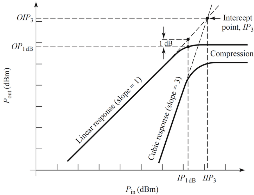
Figura 2.5: Curva teórica del punto de intercepción de tercer orden referido a la salida y del punto de compresión de 1 dB [4].
