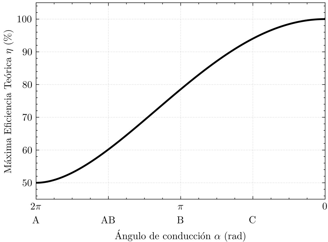
Figura 2.2: Eficiencia de drain teórica en función del ángulo de conducción, con las regiones correspondientes a las Clases A, AB, B y C señaladas.
