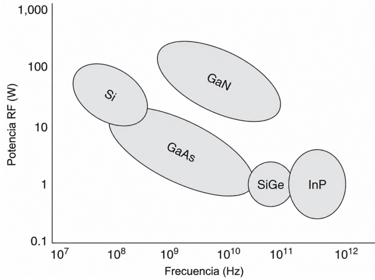
Figura 3.1: Rangos característicos de potencia de RF y frecuencia de operación alcanzables para distintas tecnologías semiconductoras [9].
