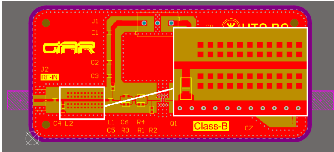
Figura 5.2: Pads adicionales incorporados para permitir la extensión de la longitud de los stubs de adaptación, en caso de requerirse ajuste experimental.
