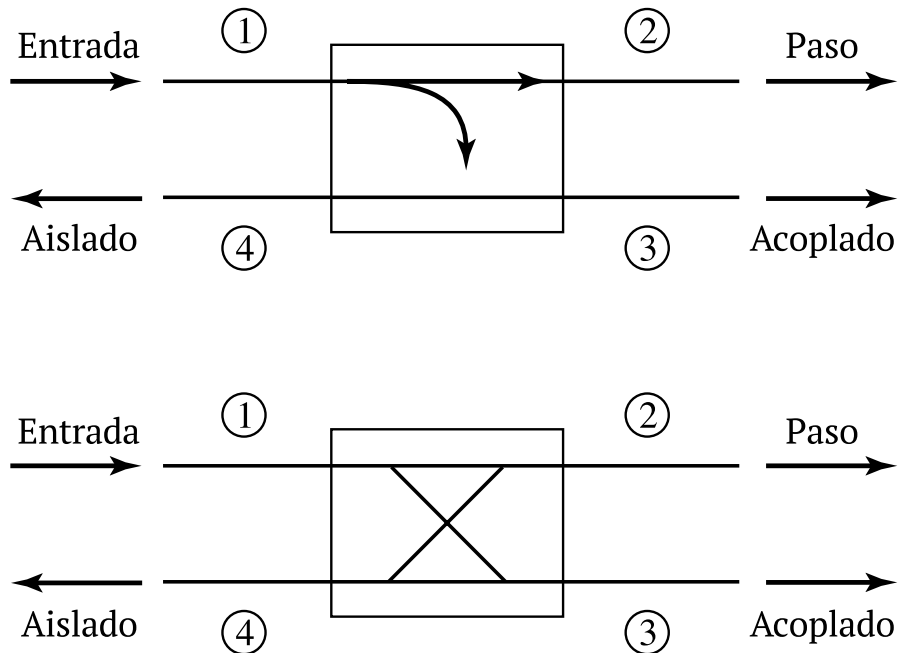
Figura 4.1: Dos símbolos comúnmente utilizados para acopladores direccionales
