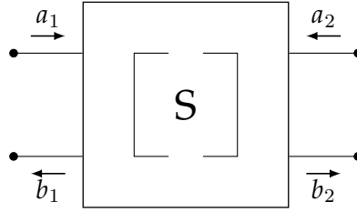
Figura 2.3: Representación simplificada de un cuadripolo mediante parámetros de dispersión ( S ).
