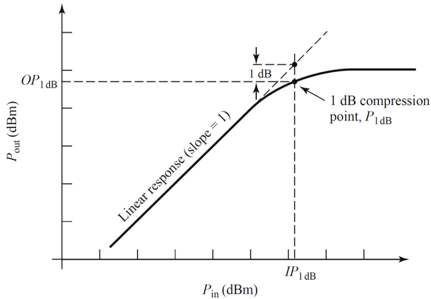
Figura 2.4: Curva teórica del punto de compresión de 1 dB [4].
