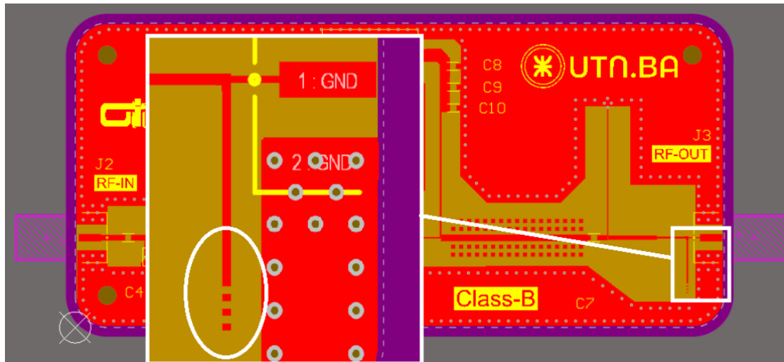
Figura 5.3: Pads adicionales incorporados para permitir la modificación del ancho de las líneas de transmisión, en caso de requerirse ajuste experimental.
