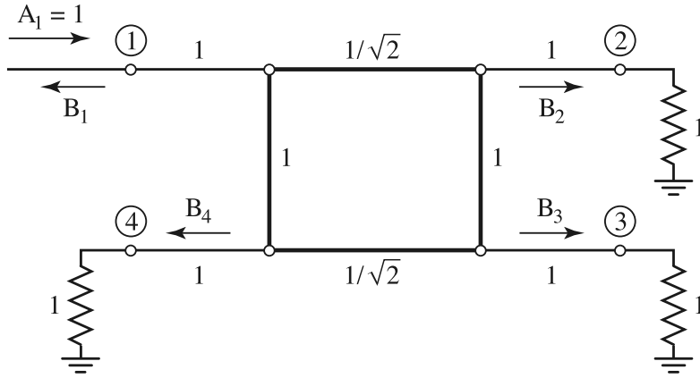
Figura 4.3: Circuito del acoplador híbrido de línea ramificada en forma normalizada.
