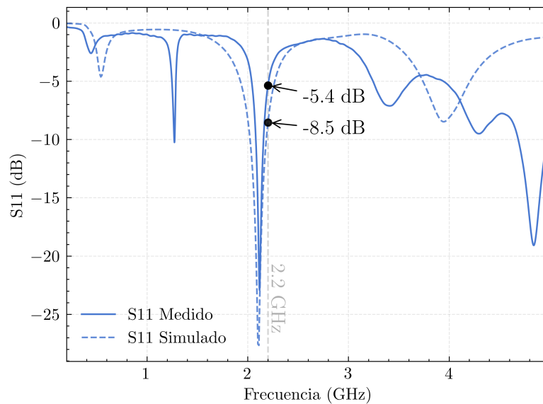
Figura 6.1: Comparación entre el S_{11} simulado (línea punteada) y medido (línea sólida) del amplificador de potencia fabricado.
