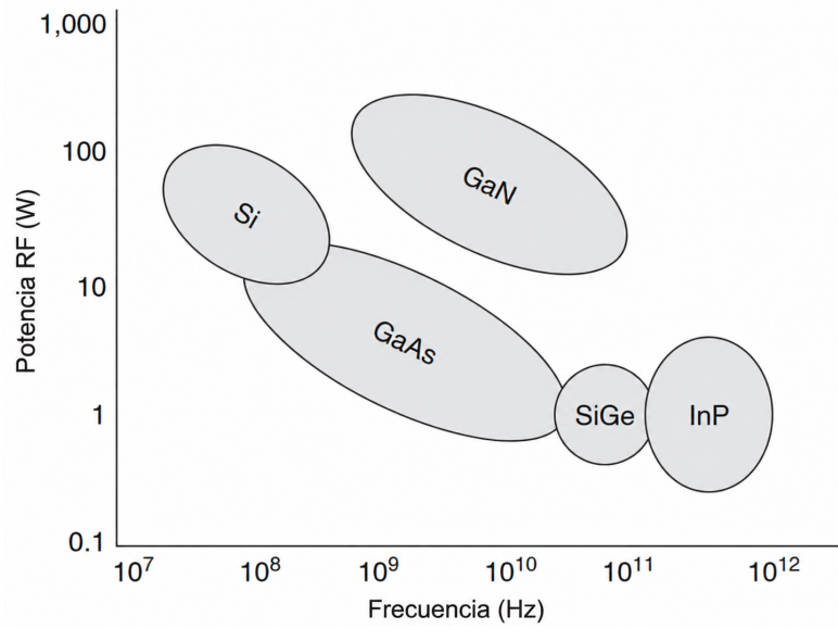
Figura 3.1: Rangos característicos de potencia de RF y frecuencia de operación alcanzables para distintas tecnologías semiconductoras [13].
