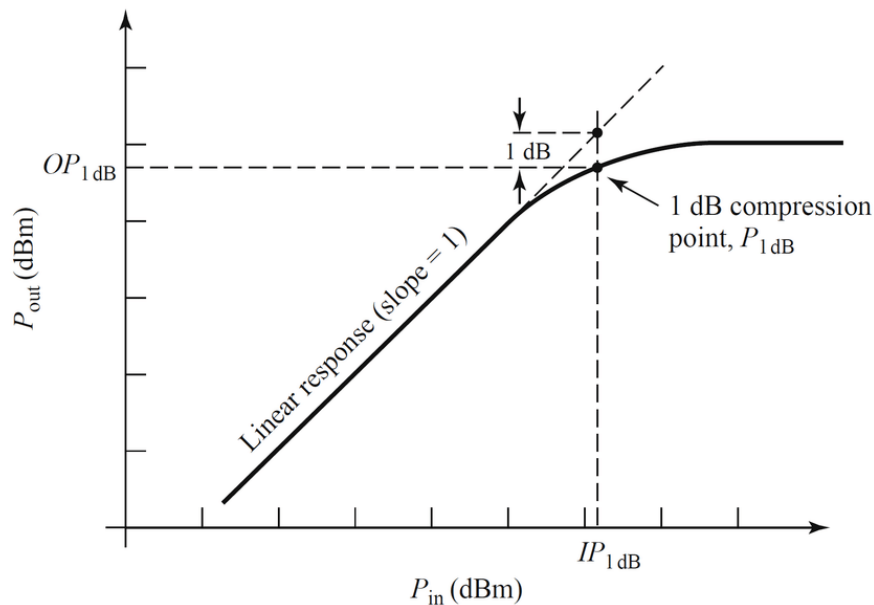
Figura 2.6: Curva teórica del punto de compresión de 1 dB [7].
