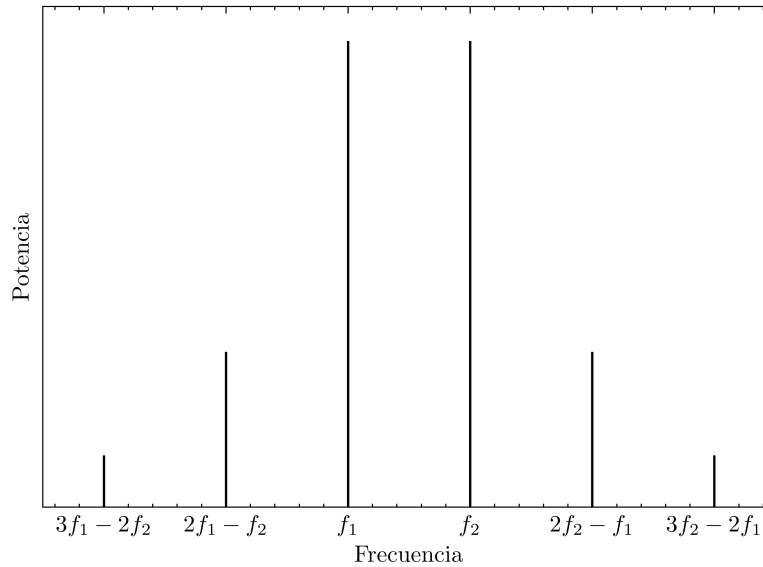
Figura 2.7: Productos de intermodulación cercanos a las frecuencias de los tonos de la señal de entrada.
