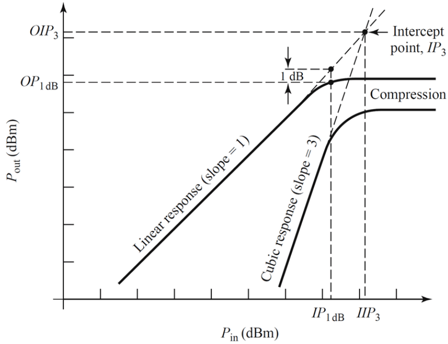
Figura 2.8: Curva teórica del punto de intersección de tercer orden referido a la salida y del punto de compresión de 1 dB [7].
