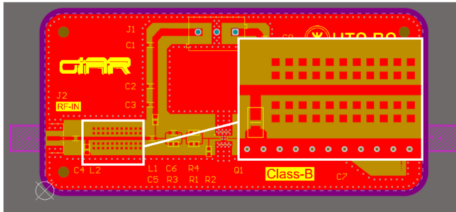
Figura 9: Pads adicionales incorporados para permitir la extensión de la longitud de los stubs de adaptación, en caso de requerirse ajuste experimental.
