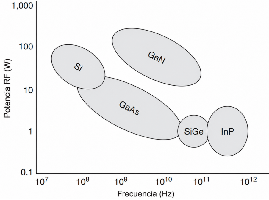
Figura 4: Rangos característicos de potencia de radiofrecuencia y frecuencia de operación alcanzables para distintas tecnologías semiconductoras [8].
