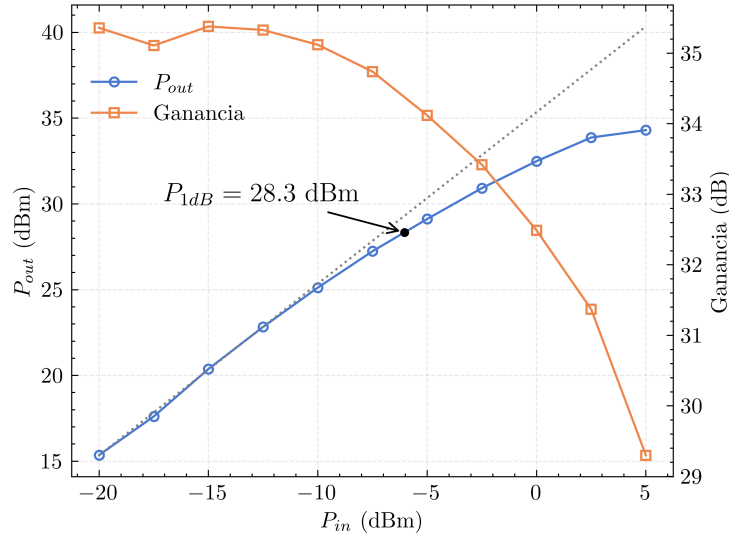
Figura 13: Potencia de salida medida (azul) y ganancia (naranja) en función de la potencia de entrada para la cadena driver-DUT. La línea punteada gris representa la característica de transferencia lineal ideal obtenida de la extrapolación de ganancia de pequeña señal.
