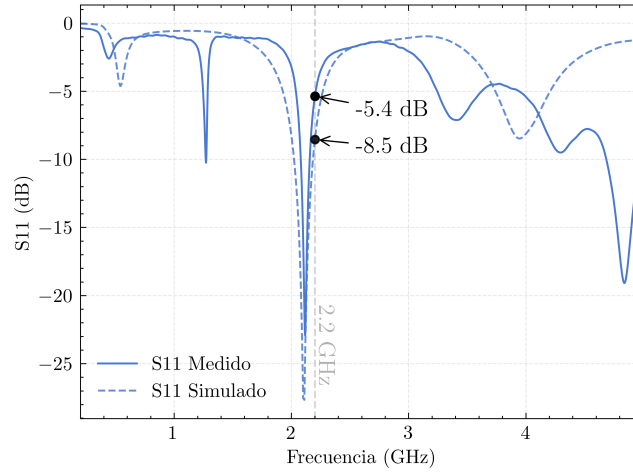
Figura 11: Comparación entre el S_{11} simulado (línea punteada) y medido (línea sólida) del amplificador de potencia fabricado.
