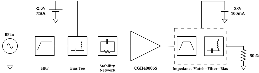
Figura 8: Diagrama en bloques de la topología propuesta para el amplificador de potencia.
