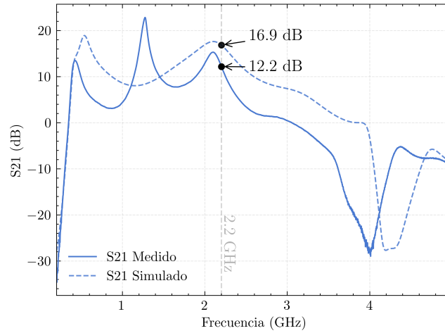
Figura 12: Comparación entre el S_{21} simulado (línea punteada) y medido (línea sólida) del amplificador de potencia fabricado.
