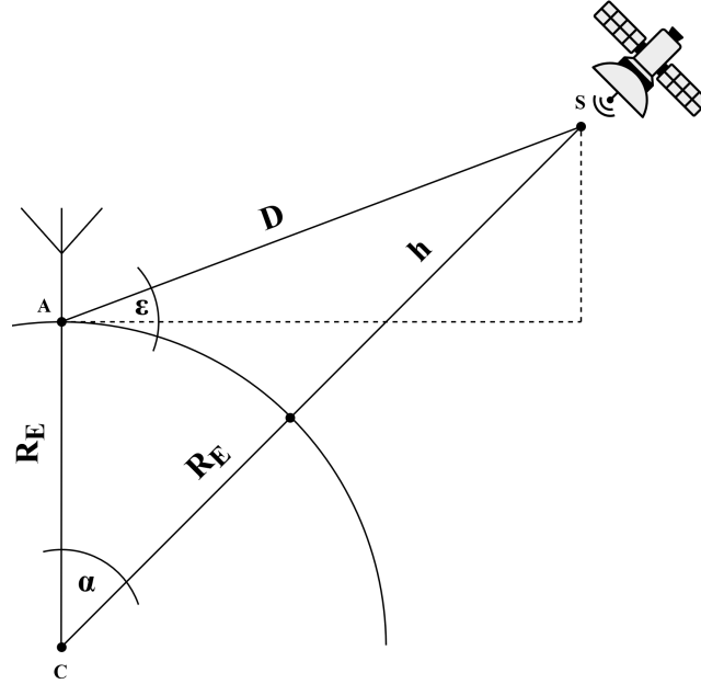
Figura 5: Modelo matemático para el cálculo de la distancia D en función del ángulo de elevación epsilon ( \epsilon ).
