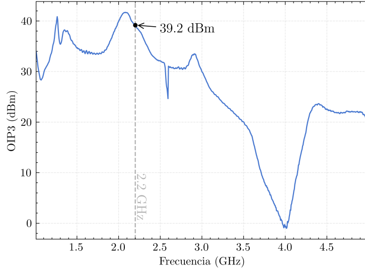
Figura 14: Barrido en frecuencia del punto de intersección de tercer orden a la salida (OIP3) medido para la cadena driver-DUT.
