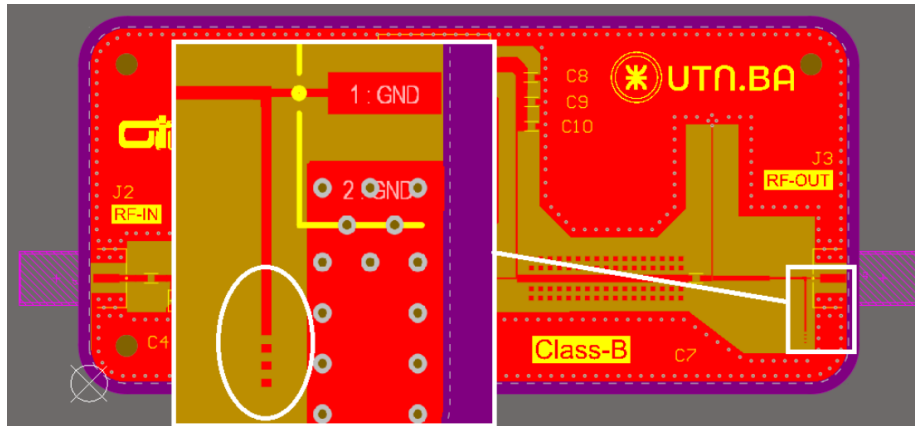
Figura 10: Pads adicionales incorporados para permitir la modificación del ancho de las líneas de transmisión, en caso de requerirse ajuste experimental.
