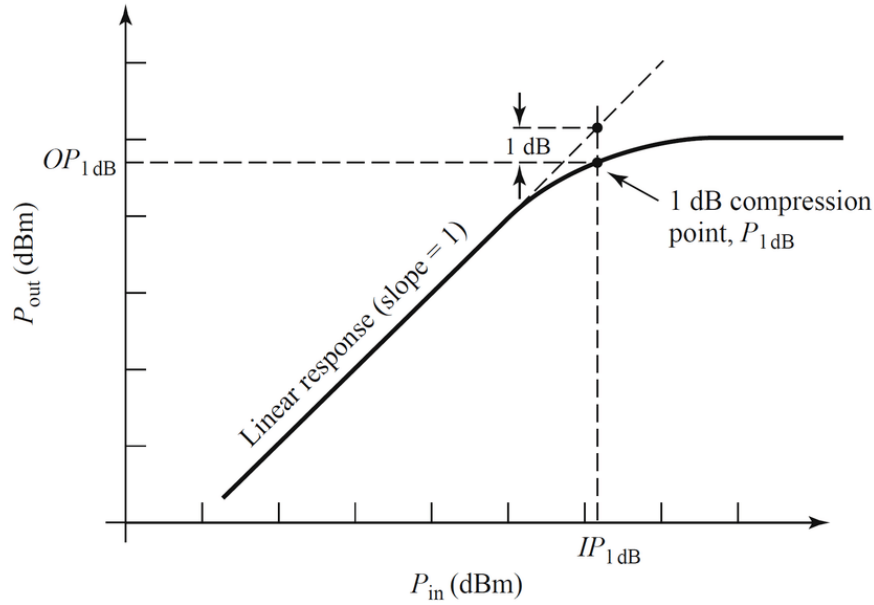
Figura 2.7: Curva teórica del punto de compresión de 1 dB [8].
