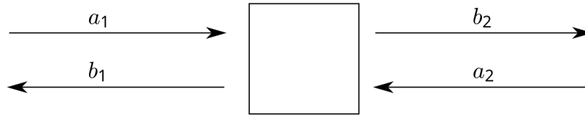
Figura 2.6: Cuadripolo genérico de dos puertos con sus ondas incidentes y reflejadas [4].
