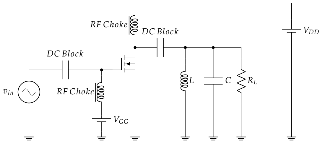
Figura 2.1: Circuito simplificado de un amplificador.
