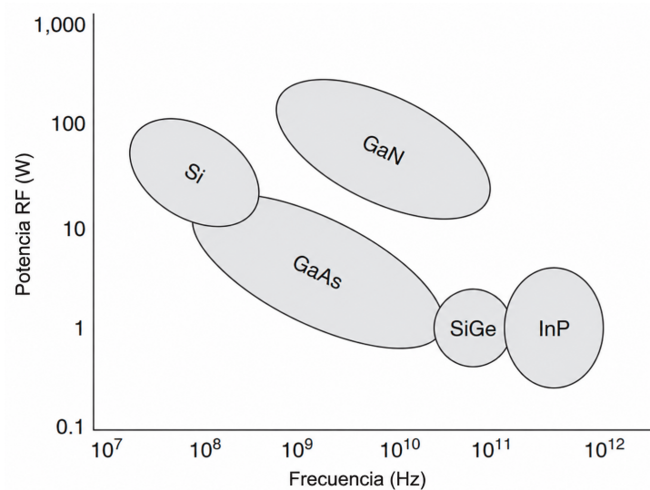
Figura 3.3: Rangos característicos de potencia de RF y frecuencia de operación alcanzables para distintas tecnologías semiconductoras [22].
