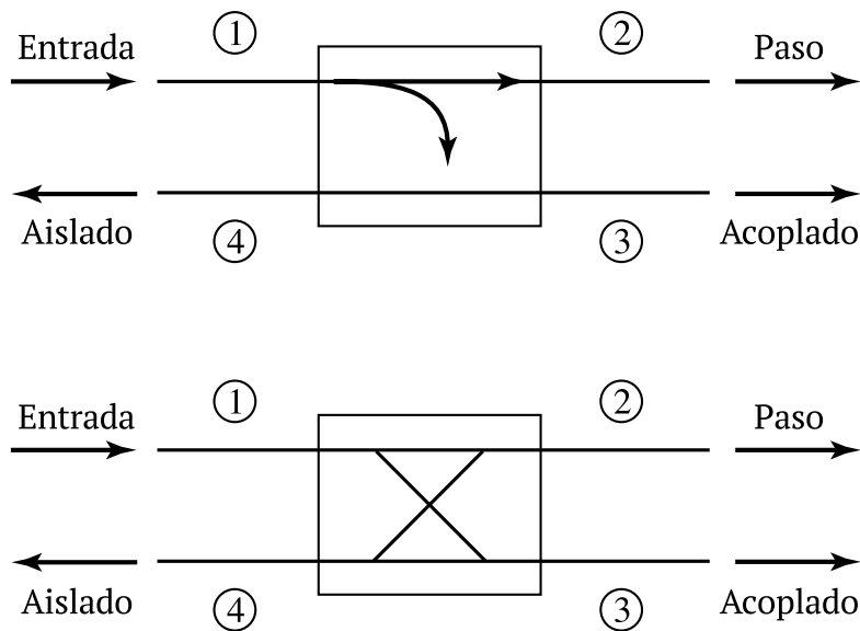
Figura 4.1: Dos símbolos comúnmente utilizados para acopladores direccionales.
