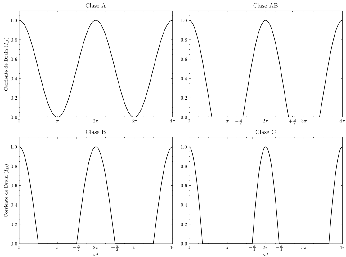
Figura 2.2: Corrientes de drain para las distintas clases de operación de un amplificador suponiendo la debida polarización del circuito para cada caso.
