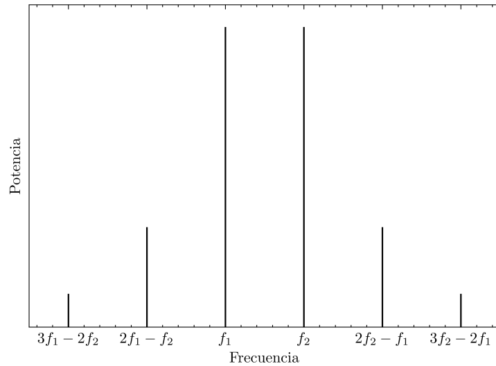
Figura 2.8: Productos de intermodulación cercanos a las frecuencias de los tonos de la señal de entrada.
