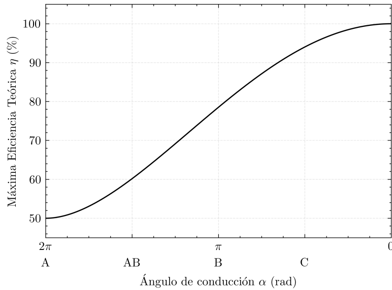
Figura 2.4: Eficiencia de drain teórica en función del ángulo de conducción, con las regiones correspondientes a las Clases A, AB, B y C señaladas.
