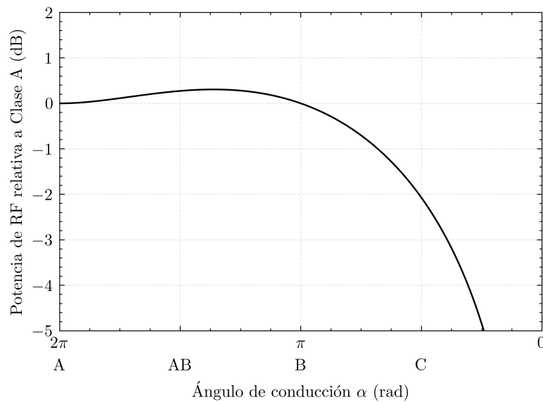
Figura 2.5: Potencia de RF entregada a la carga, relativa a Clase A, en función del ángulo de conducción, asumiendo carga óptima y cortocircuito en las frecuencias armónicas.
