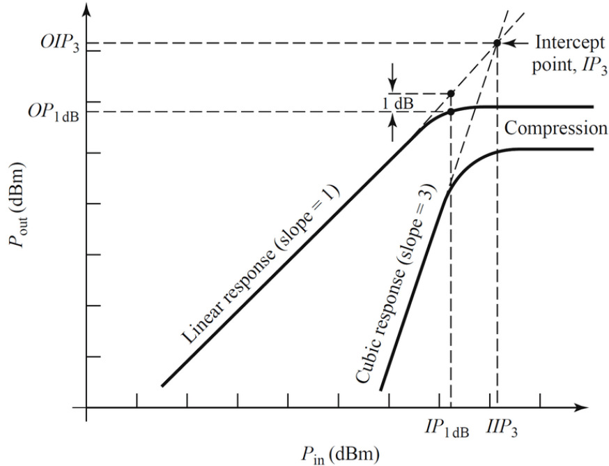
Figura 2.9: Curva teórica del punto de intercepción de tercer orden referido a la salida y del punto de compresión de 1 dB [8].
