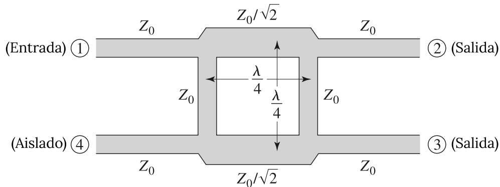
Figura 4.2: Geometría de un acoplador de línea ramificada.
