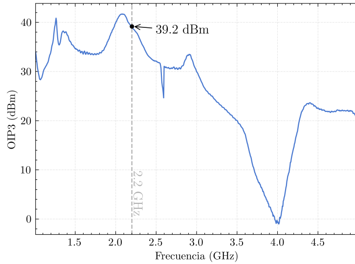
Figura 14: Barrido en frecuencia del punto de intercepción de tercer orden a la salida (OIP3) medido para la cadena driver-DUT.
