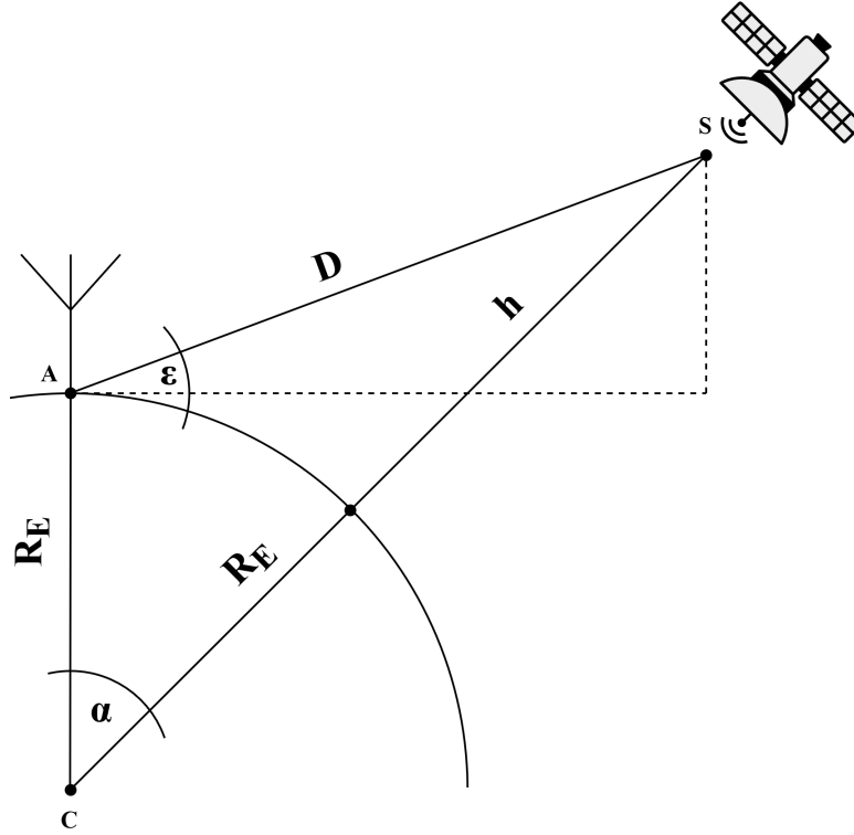
Figura 7.12: Modelo matemático para el cálculo de la distancia D en función del ángulo de elevación \epsilon ( \epsilon ).
