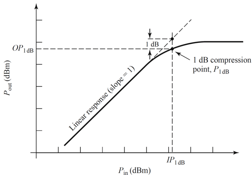
Figura 2.6: Curva teórica del punto de compresión de 1 dB [6].
