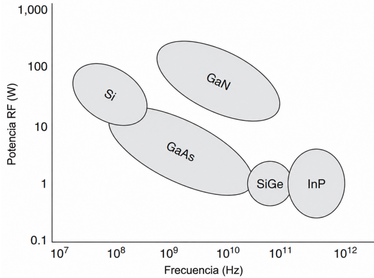
Figura 3.1: Rangos característicos de potencia de RF y frecuencia de operación alcanzables para distintas tecnologías semiconductoras [11].
