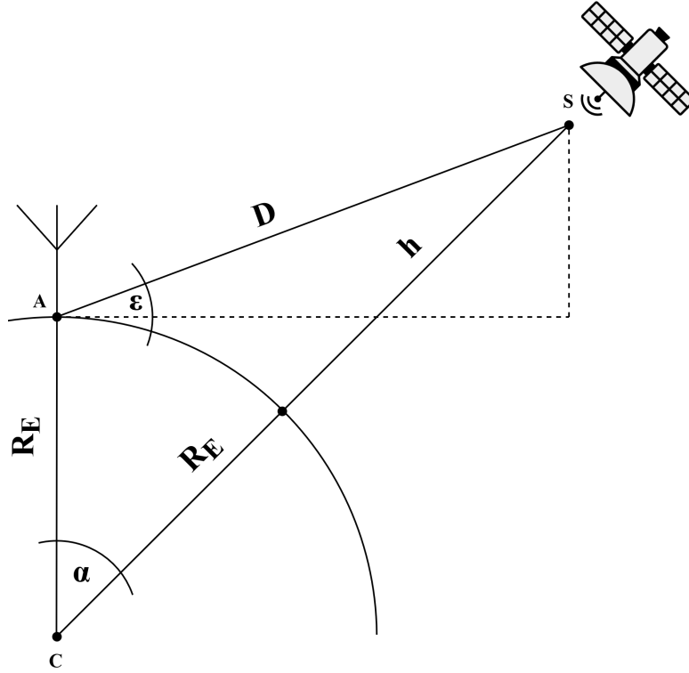
Figura 5.4: Modelo matemático para el cálculo de la distancia D en función del ángulo de elevación \epsilon ( \epsilon ).
