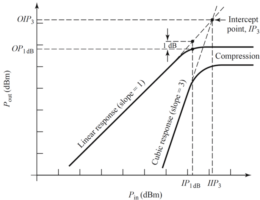
Figura 2.7: Curva teórica del punto de intercepción de tercer orden referido a la salida y del punto de compresión de 1 dB [6].
