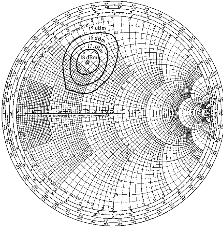
Figura 2.9: Diagrama de Smith con contornos de impedancias para distintos valores de potencia de salida constante en un transistor de potencia[6, p. 598].
