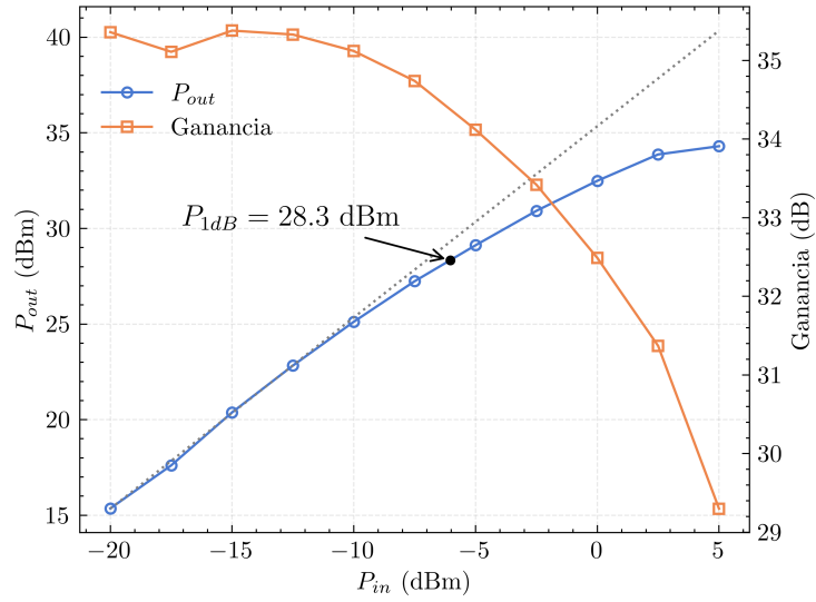
Figura 14: Potencia de salida medida (azul) y ganancia (naranja) en función de la potencia de entrada para la cadena driver-DUT. La línea punteada gris representa la característica de transferencia lineal ideal obtenida de la extrapolación de ganancia de pequeña señal.
