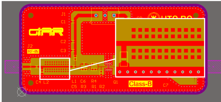
Figura 10: Pads adicionales incorporados para permitir la extensión de la longitud de los stubs de adaptación, en caso de requerirse ajuste experimental.
