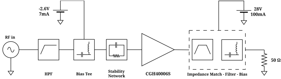
Figura 9: Diagrama en bloques de la topología propuesta para el amplificador de potencia.
