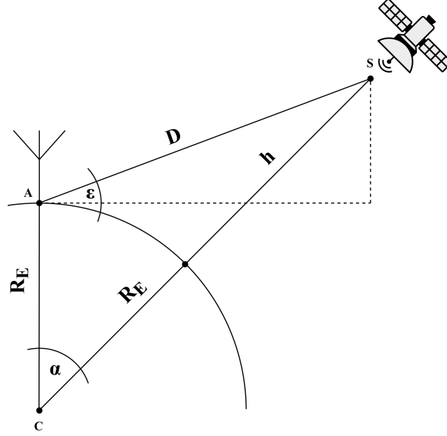
Figura 6: Modelo matemático para el cálculo de la distancia D en función del ángulo de elevación epsilon ( \epsilon ).
