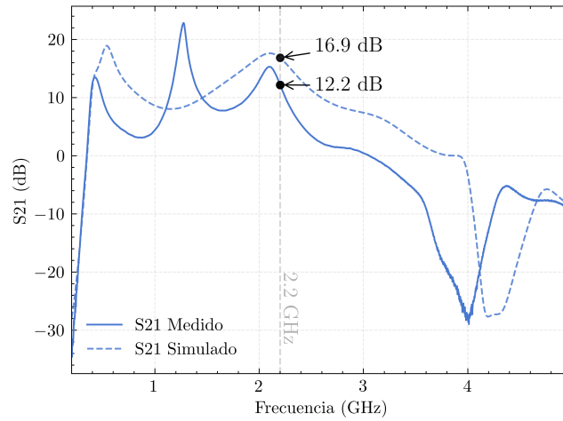
Figura 13: Comparación entre el S_{21} simulado (línea punteada) y medido (línea sólida) del amplificador de potencia fabricado.
