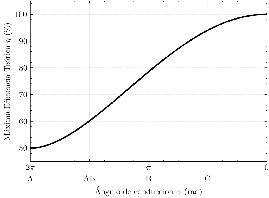
Figura 3: Eficiencia de drain teórica en función del ángulo de conducción, con las regiones correspondientes a las Clases A, AB, B y C señaladas.
