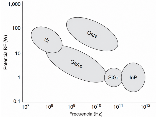
Figura 5: Rangos característicos de potencia de RF y frecuencia de operación alcanzables para distintas tecnologías semiconductoras [8].
