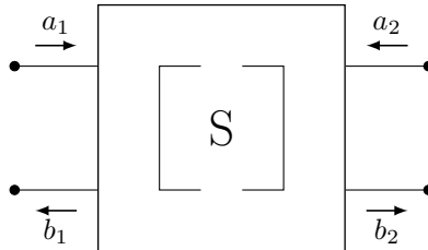
Figura 4: Representación simplificada de un cuadripolo mediante parámetros de dispersión ( S ).
