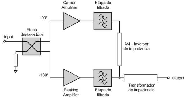
Figura 1: Diagrama en bloques de la topología Doherty.
