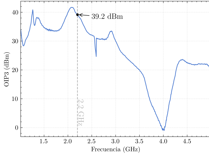
Figura 15: Barrido en frecuencia del punto de intercepción de tercer orden a la salida (OIP3) medido para la cadena driver-DUT.
