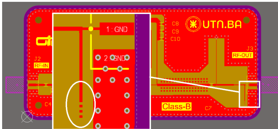
Figura 11: Pads adicionales incorporados para permitir la modificación del ancho de las líneas de transmisión, en caso de requerirse ajuste experimental.
