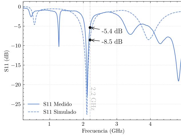
Figura 12: Comparación entre el S_{11} simulado (línea punteada) y medido (línea sólida) del amplificador de potencia fabricado.
