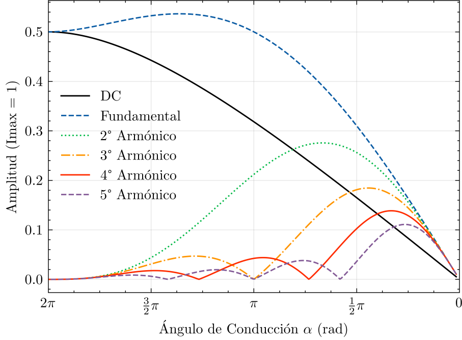
Figura 2: Amplitud normalizada de las componentes I_{dc} a I_5 de la corriente de drain en función del ángulo de conducción \alpha .
