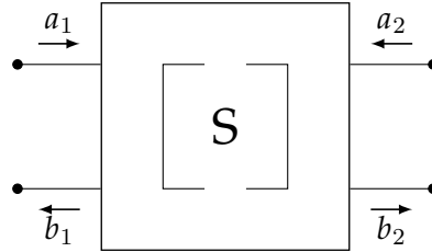
Figura 2.3: Representación simplificada de un cuadripolo mediante parámetros de dispersión ( S ).
