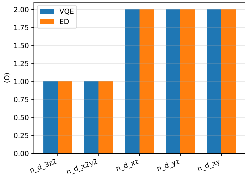
Per d-orbital occupation
