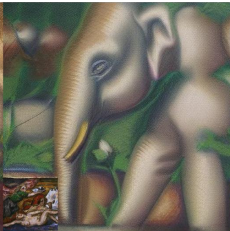
V2 adain_2blk
