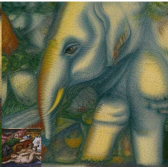
V7 proc05_adain
