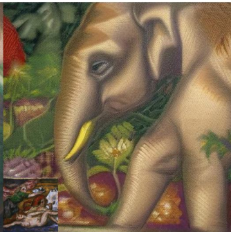
V4 no_adain_2blk
