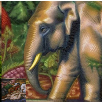
V3 no_adain_1blk
