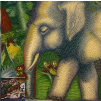
V6 proc05_no_adain
