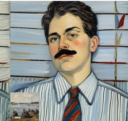
V7 proc05_adain
