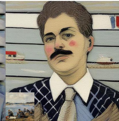
V4 no_adain_2blk
