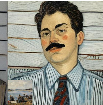
V6 proc05_no_adain
