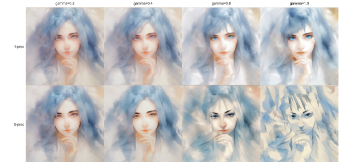
图 11. 在采用AdaIN的 up_blocks.0.attentions.1 内1个与5个self-attention processor配置在不同 \gamma 值下的风格迁移效果对比。上行为1-processor StyleKV配置，下行为5-processor StyleKV配置（本文方法）。更多目标processor带来更强的风格注入（下行风格纹理更明显），在展示样例中仍能保持较好的内容结构。
