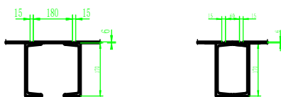
炉皮钢板焊接详图 1:20
