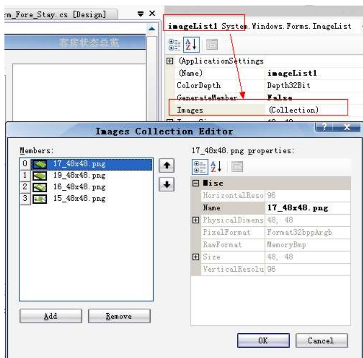
图 3 imageList1 控件属性设置
