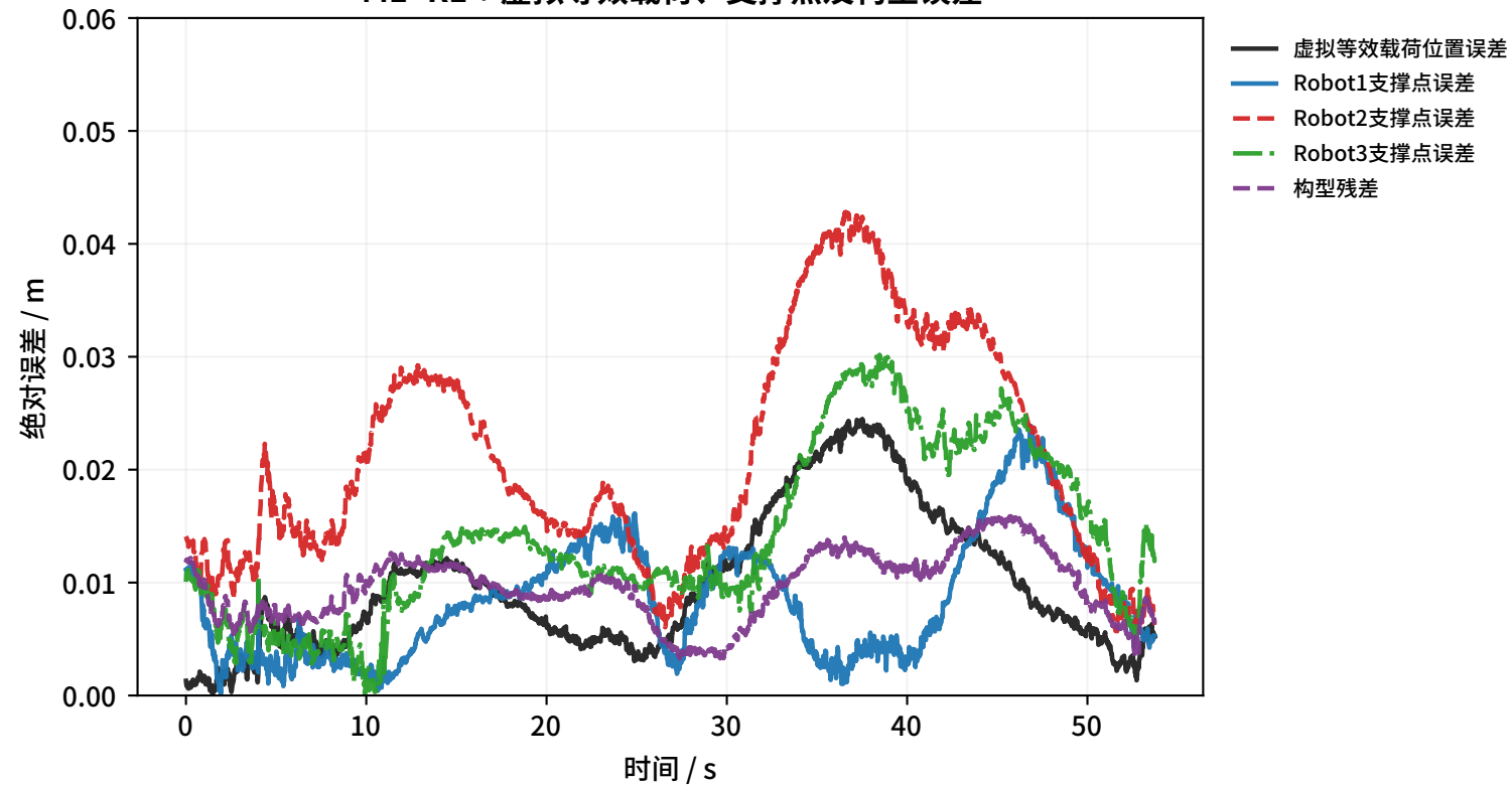
M1+R1：虚拟等效载荷、支撑点及构型误差
