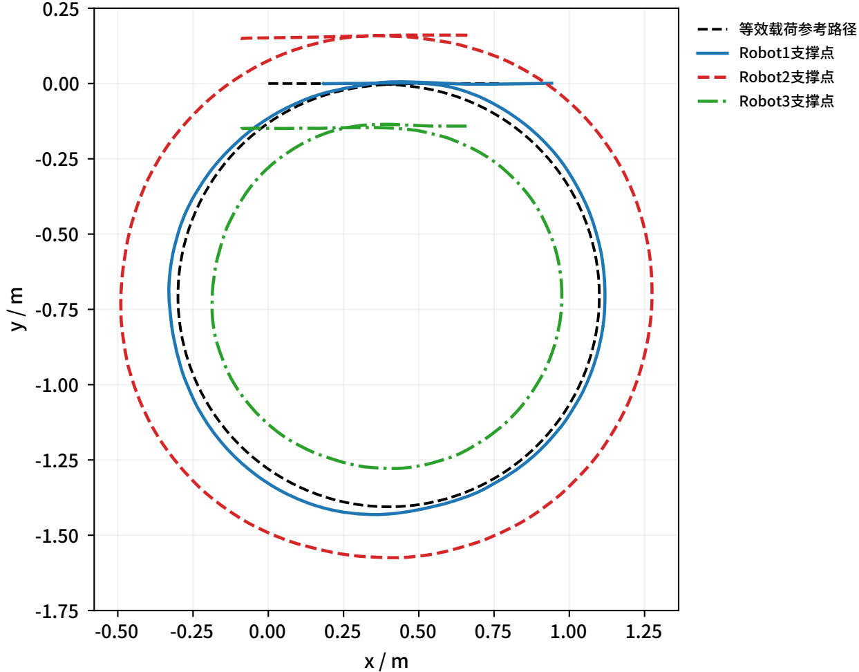
本文算法组（Robot2降额）：R=0.7m顺时针圆形路径
