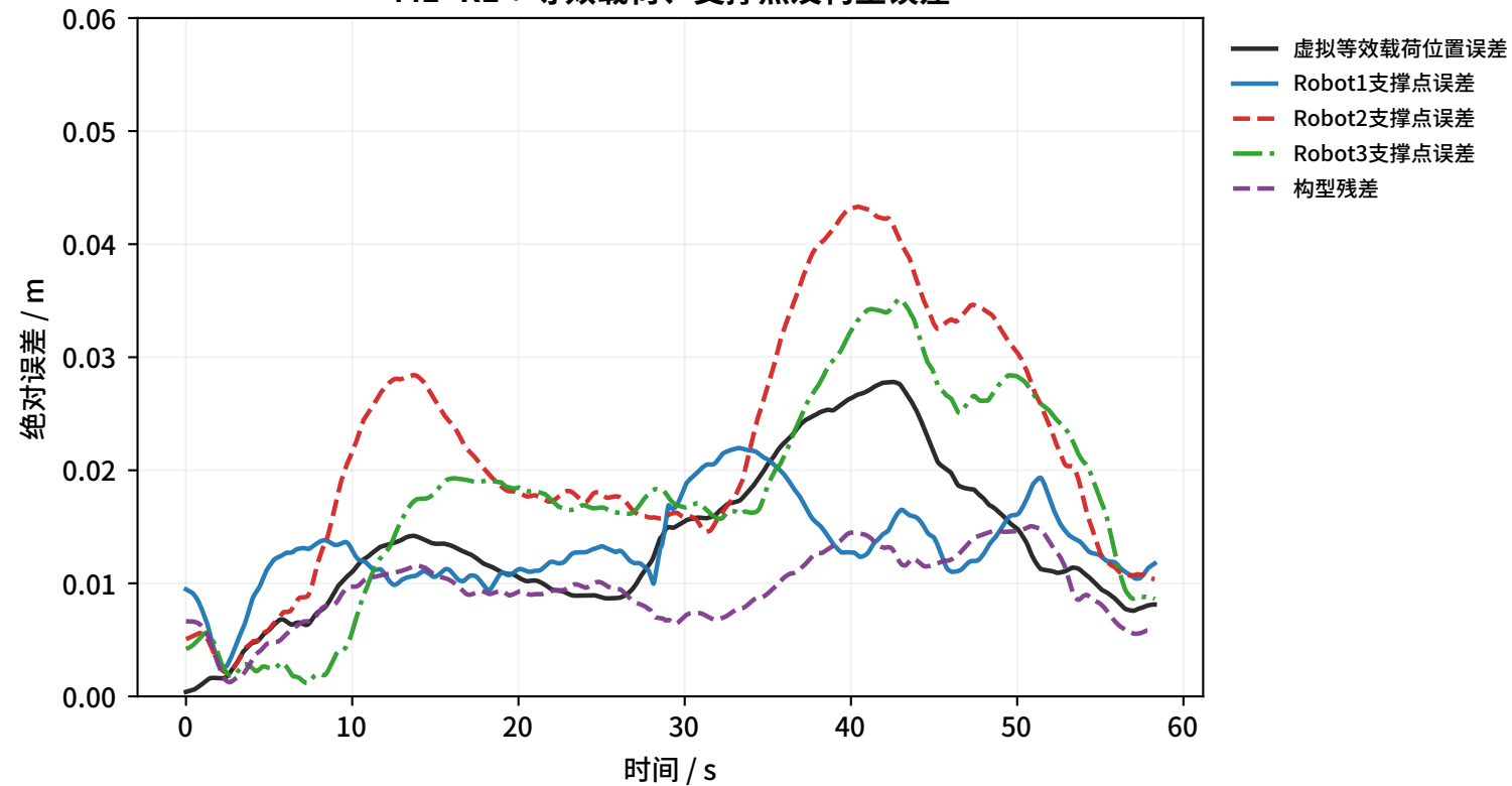
M1+R1：等效载荷、支撑点及构型误差
