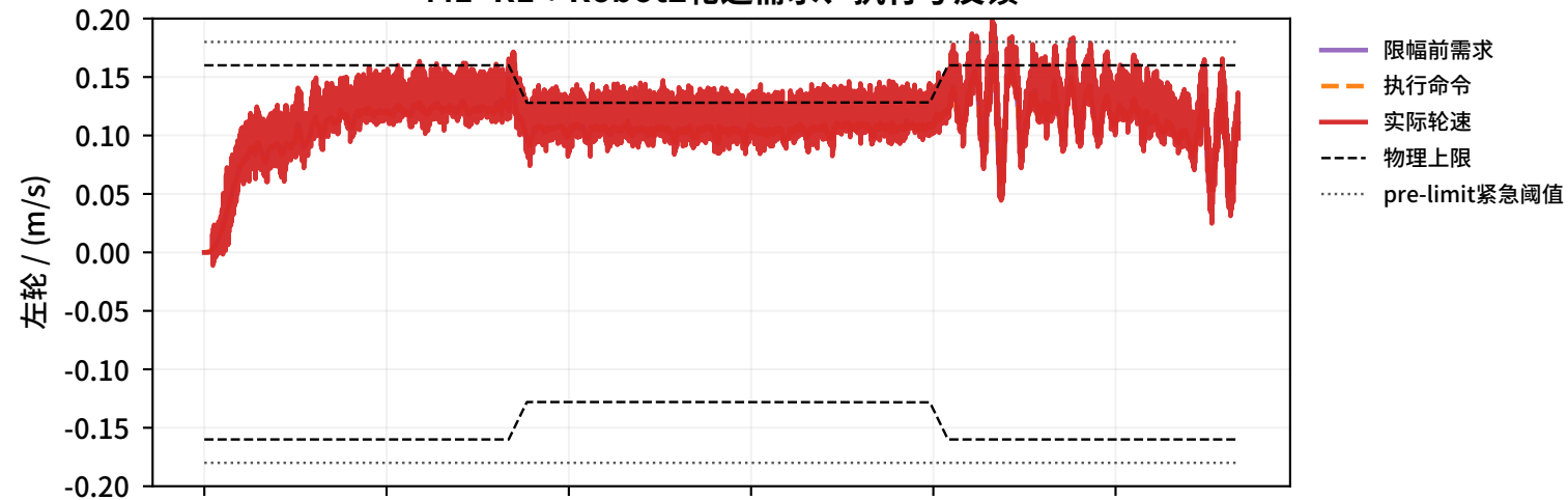
M1+R1：Robot2轮速需求、执行与反馈
