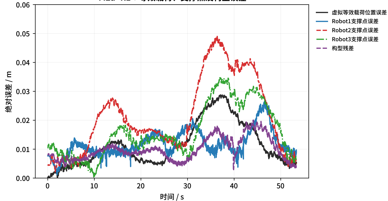
M2a+R1：等效载荷、支撑点及构型误差
