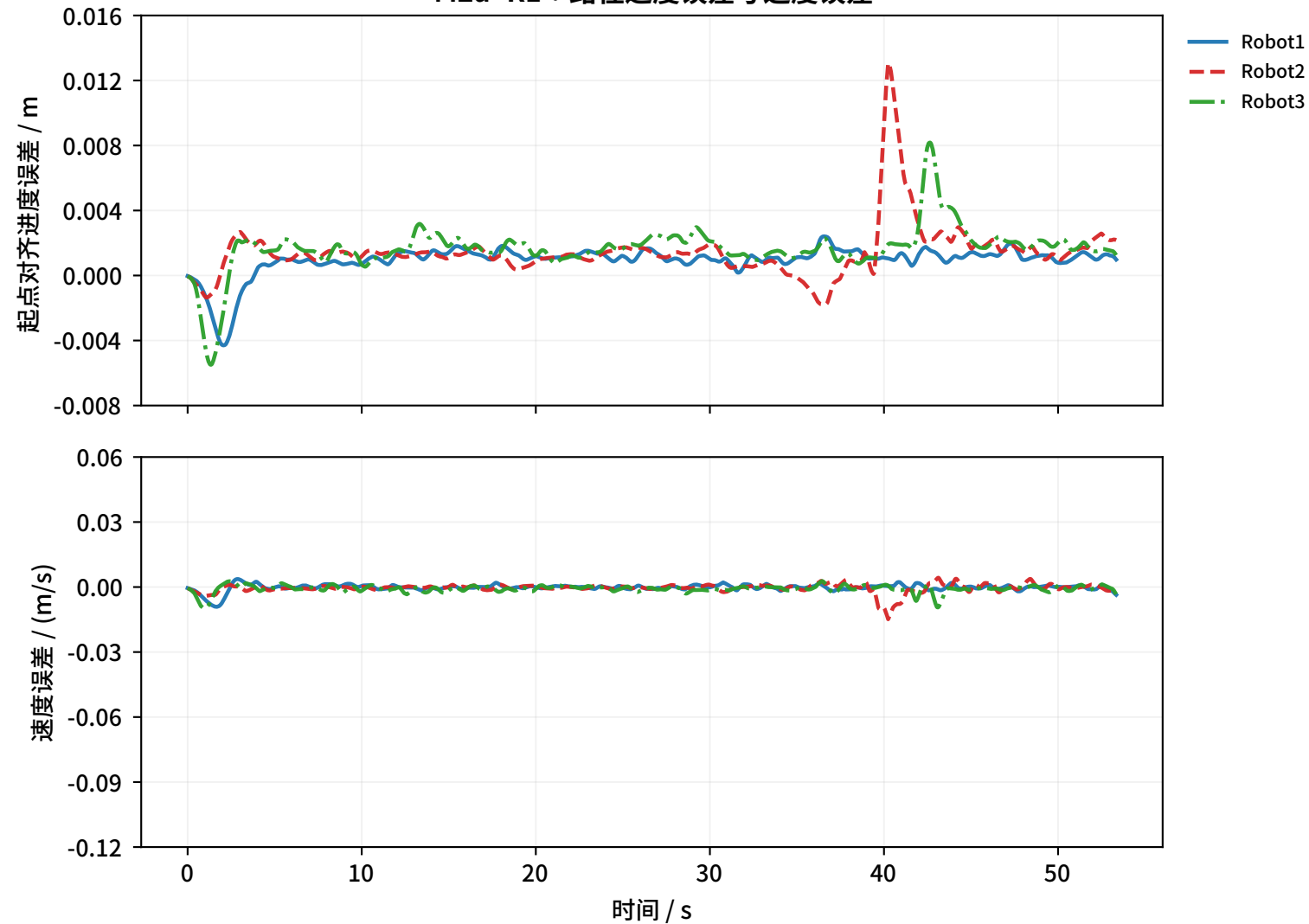
M2a+R1：路径进度误差与速度误差
