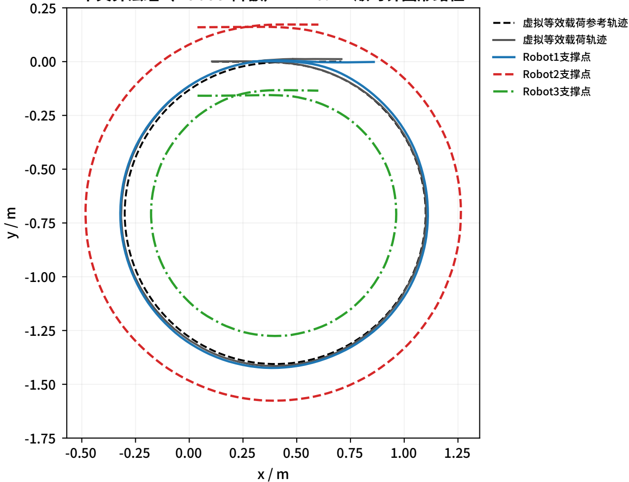
本文算法组 (Robot2降额) : R=0.7\text{m} 顺时针圆形路径
