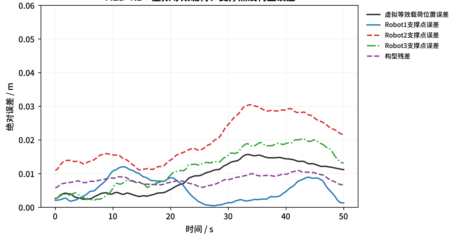
M2a+R1：虚拟等效载荷、支撑点及构型误差
