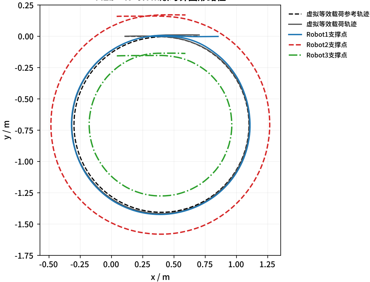
M2b : R=0.7m顺时针圆形路径
