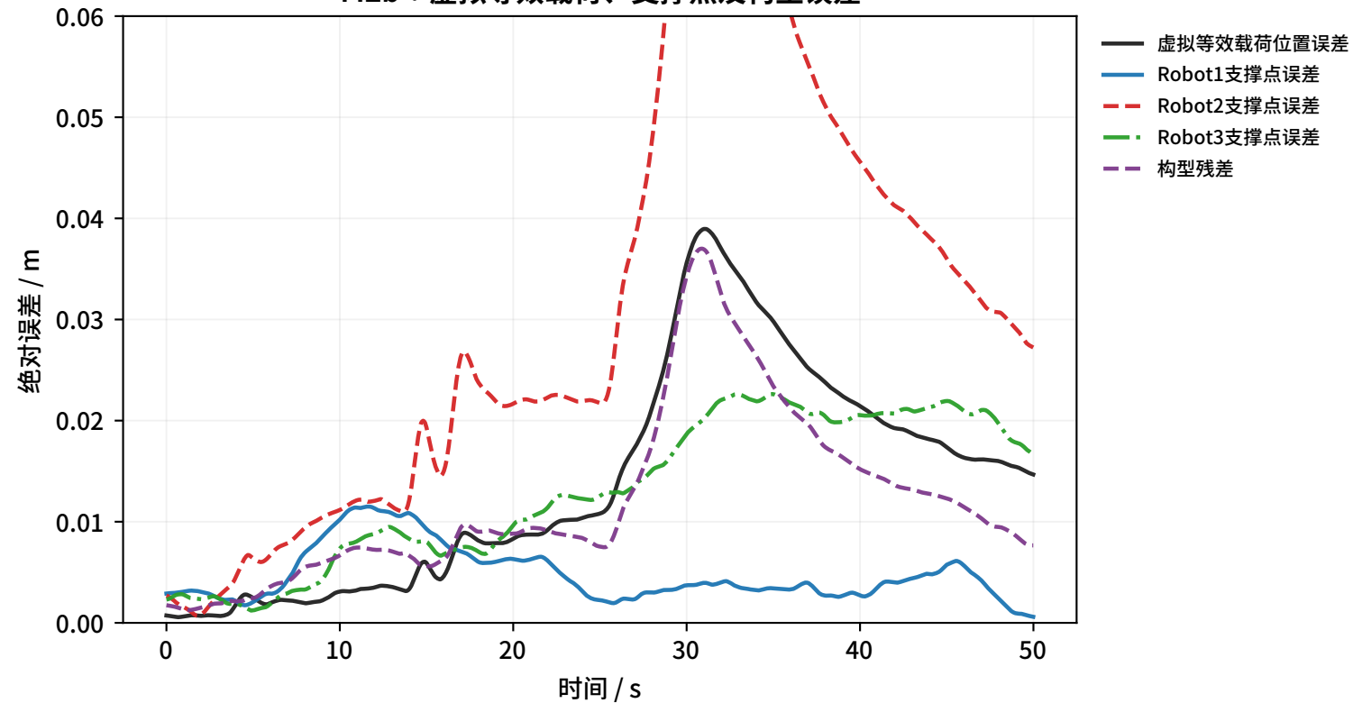
M2b：虚拟等效载荷、支撑点及构型误差
