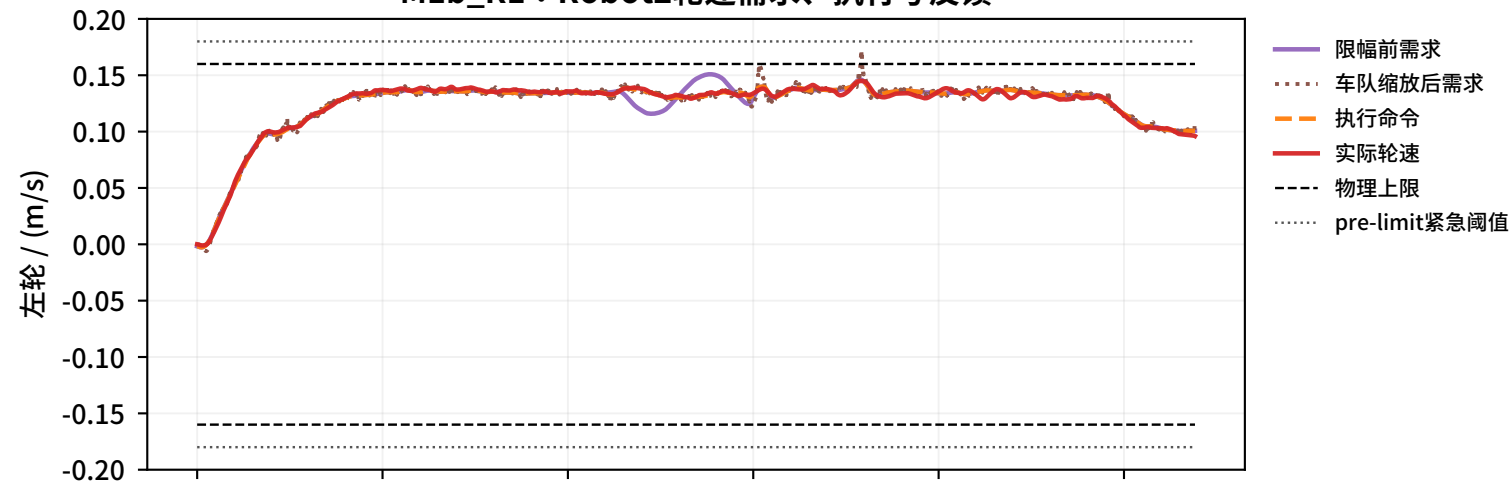
M1b_R1 : Robot2轮速需求、执行与反馈
