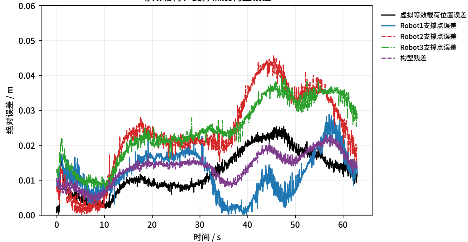
等效载荷、支撑点及构型误差
