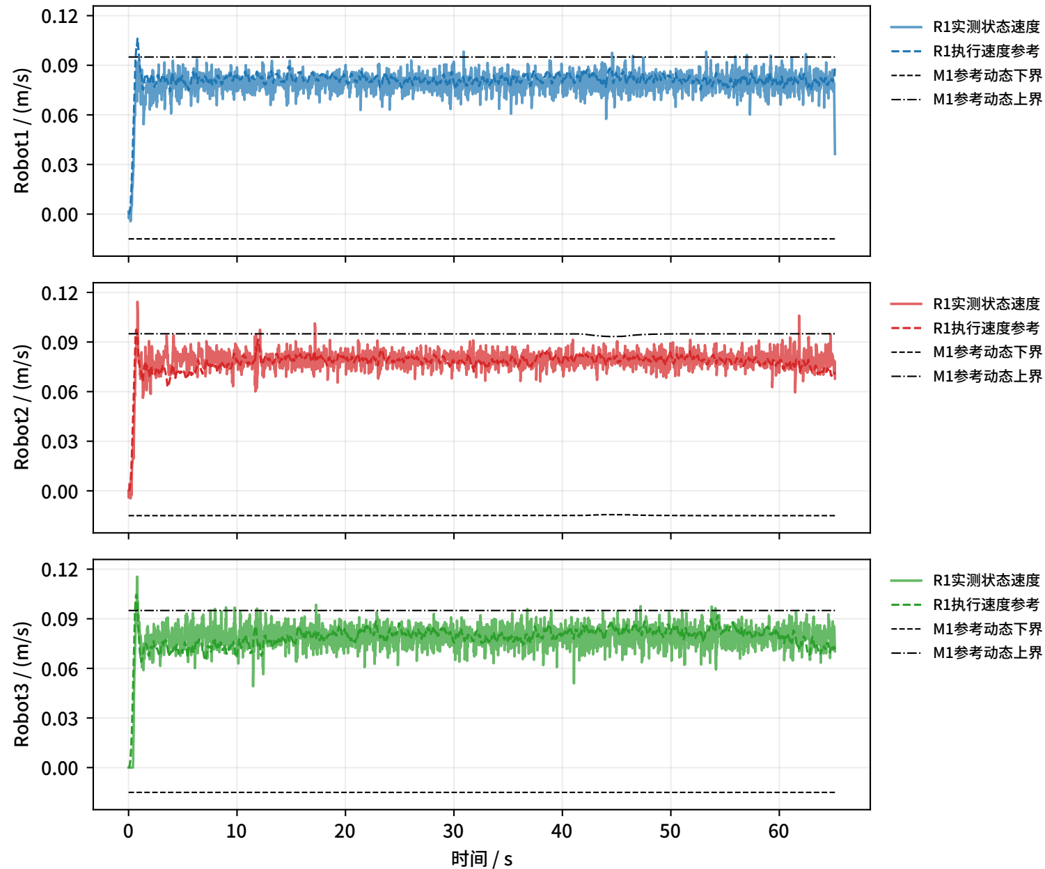
M1参考动态边界与R1执行/实测速度（语义分离）
