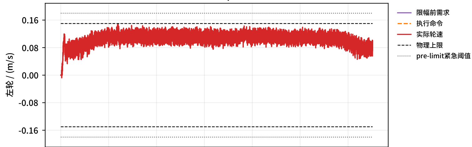
Robot2轮速执行链（物理限幅与pre-limit紧急阈值语义分离）
