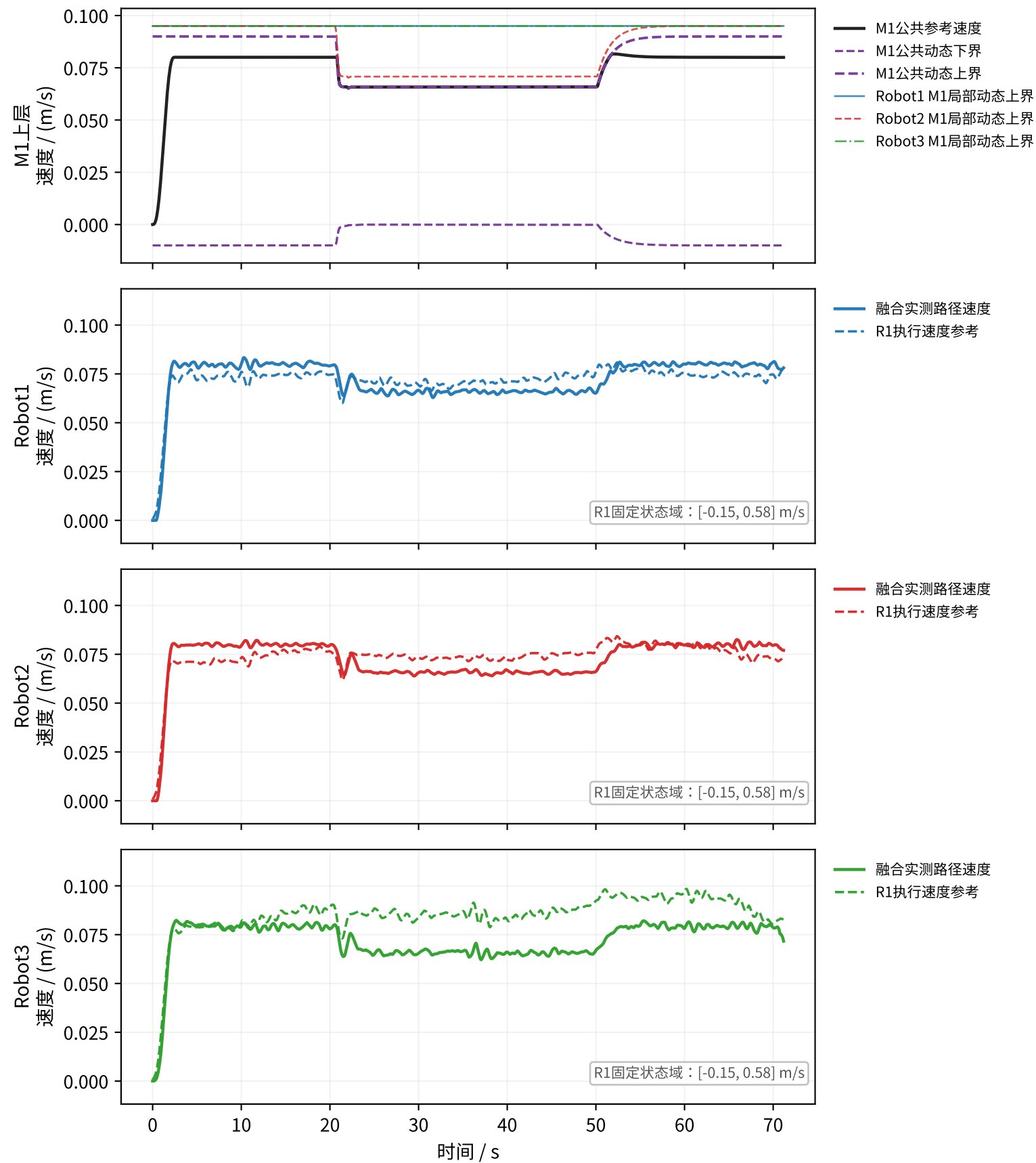
M1+R1：M1上层参考约束与R1下层执行跟踪
