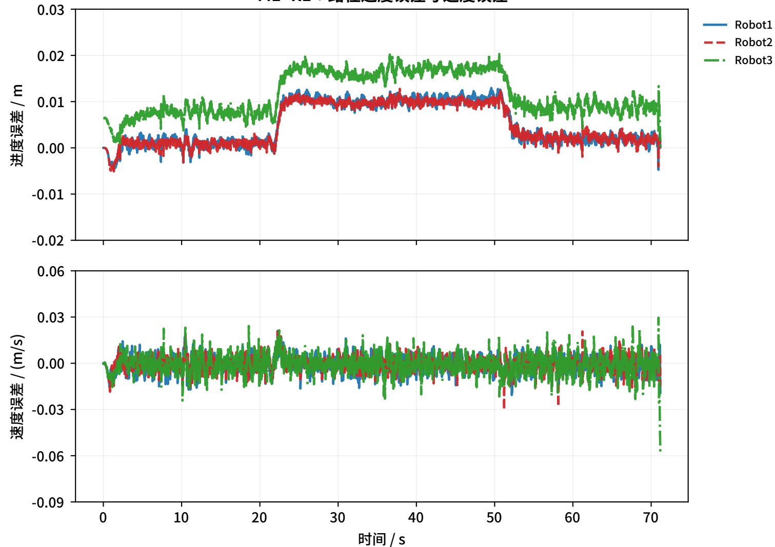
M1+R1：路径进度误差与速度误差
