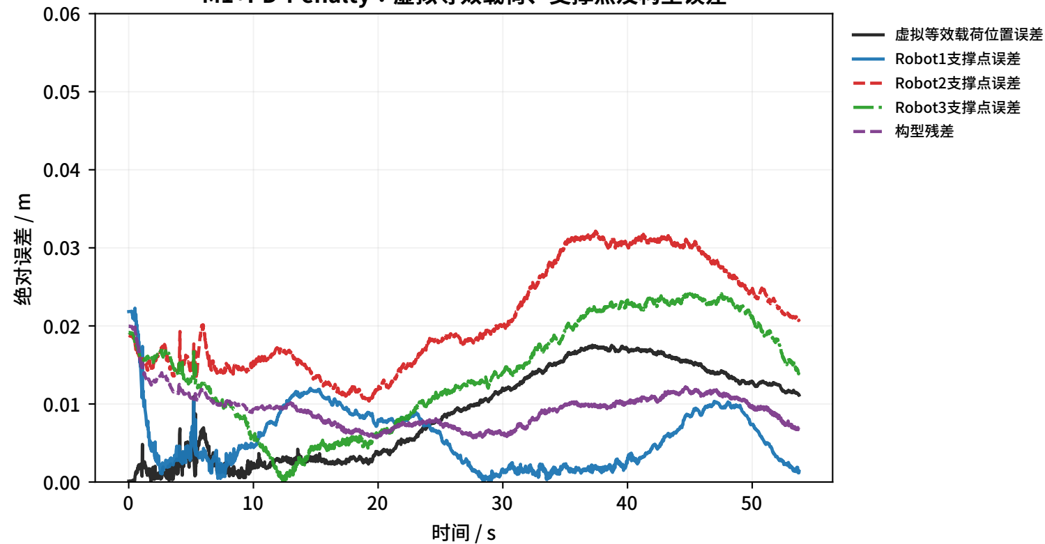
M1+PD-Penalty：虚拟等效载荷、支撑点及构型误差
