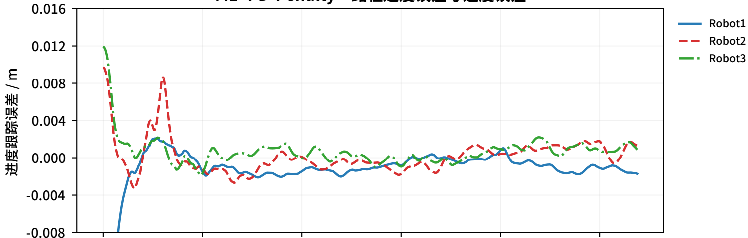
M1+PD-Penalty：路径进度误差与速度误差
