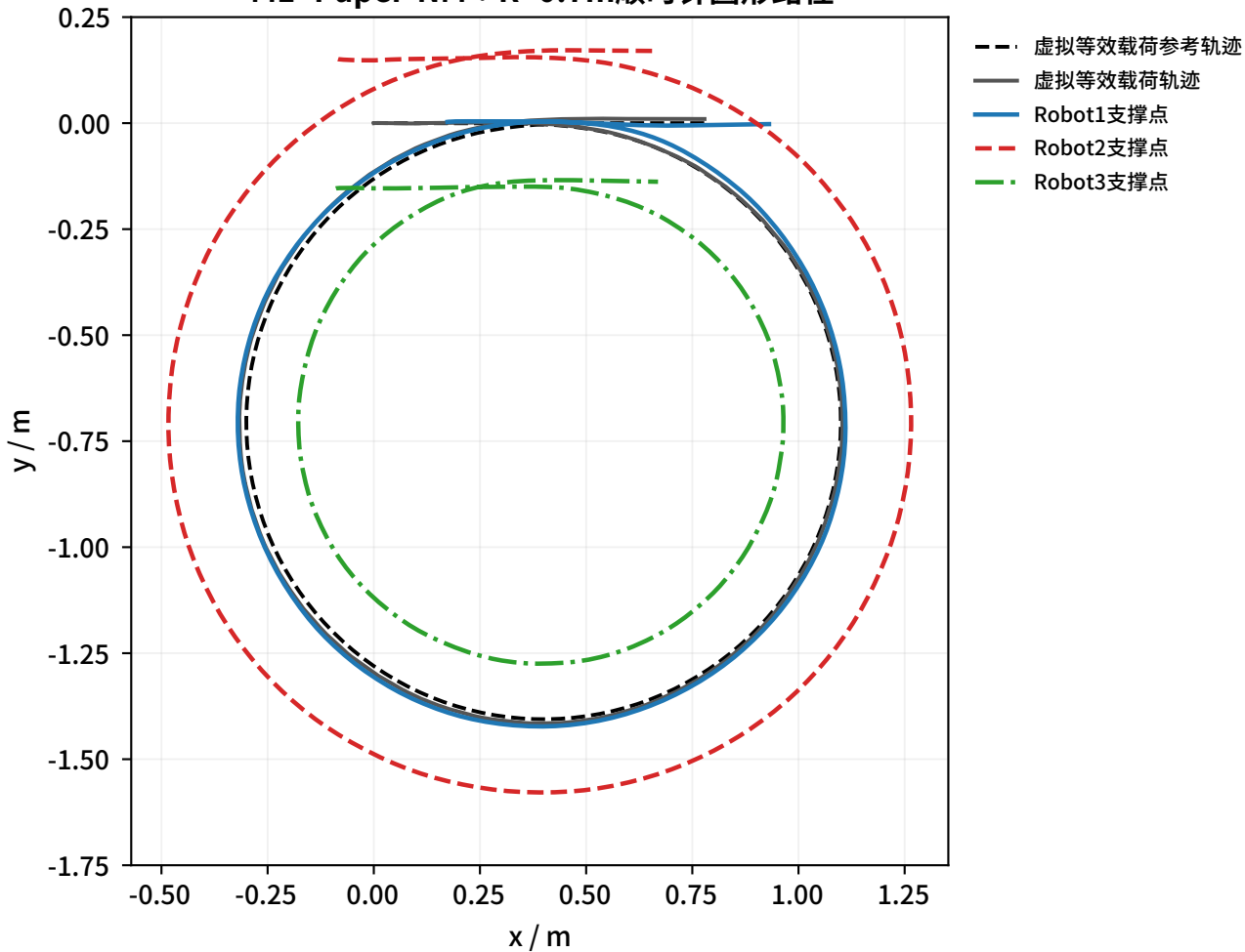
M1+Paper-NM : R=0.7m顺时针圆形路径
