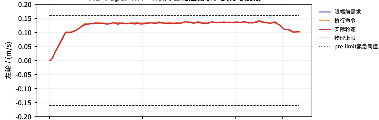
M1+Paper-NM : Robot2轮速需求、执行与反馈
