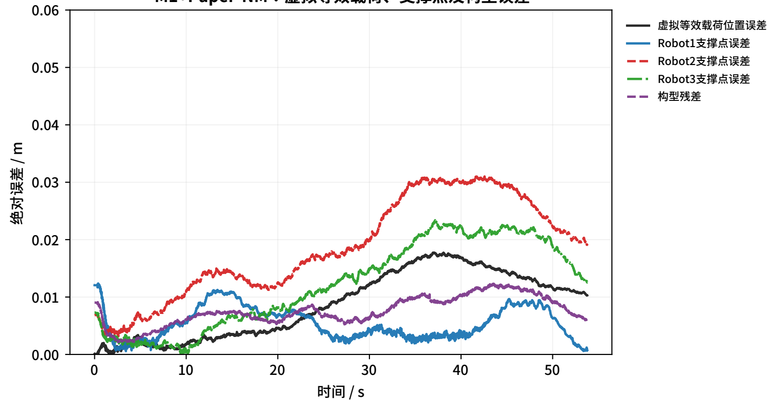
M1+Paper-NM：虚拟等效载荷、支撑点及构型误差
