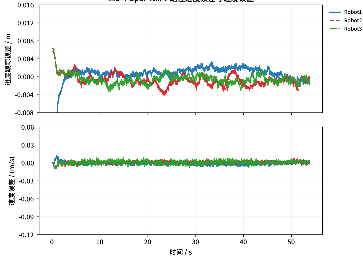
M1+Paper-NM：路径进度误差与速度误差
