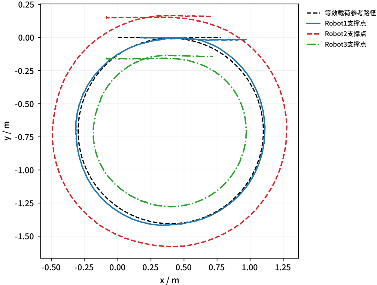
冻结工程基线：R=0.7 m顺时针圆形路径（平滑进出）与三车支撑点轨迹
