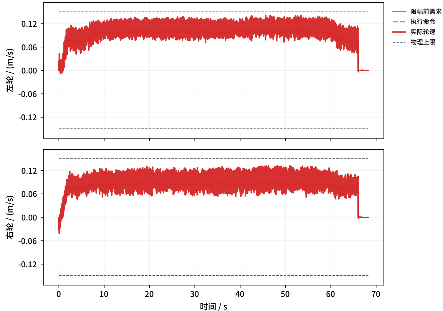
冻结工程基线：Robot2轮速需求、执行与反馈
