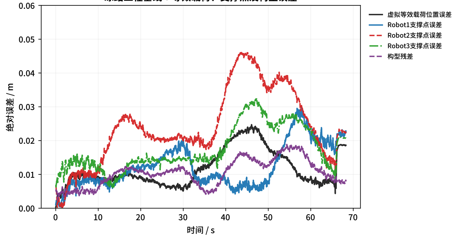
冻结工程基线：等效载荷、支撑点及构型误差
